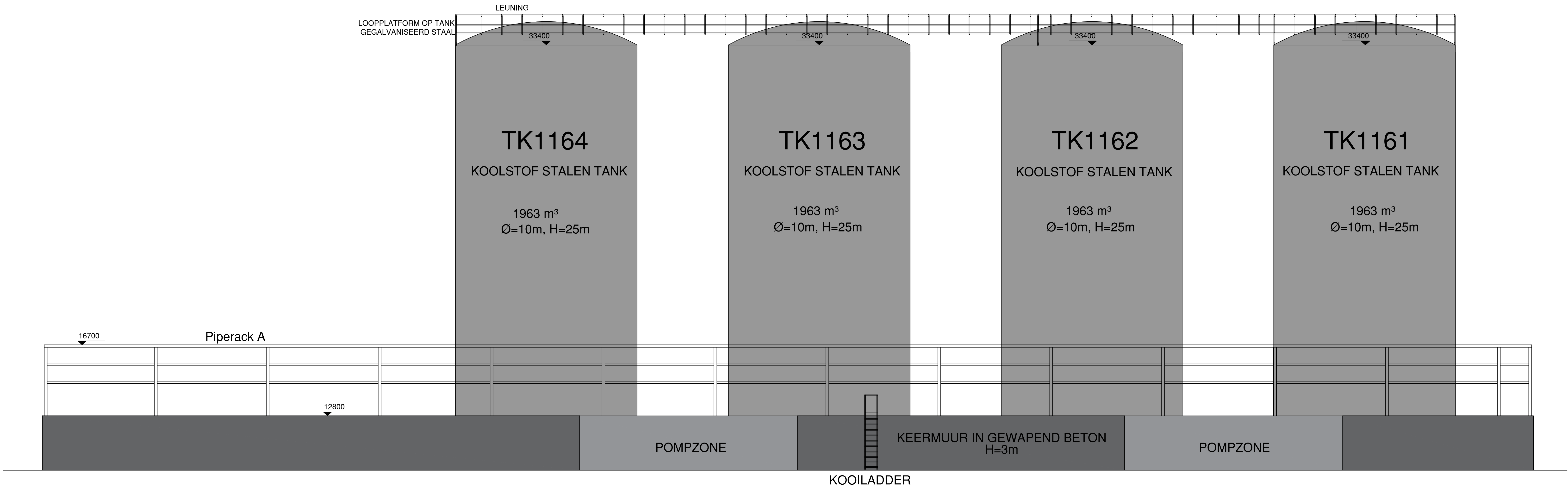
Aanzicht oost
