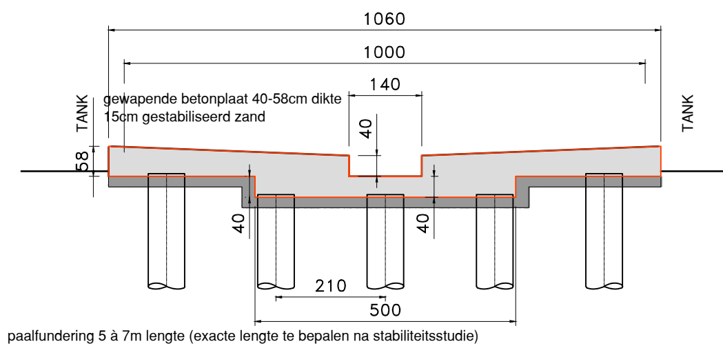
SNEDE A-A
