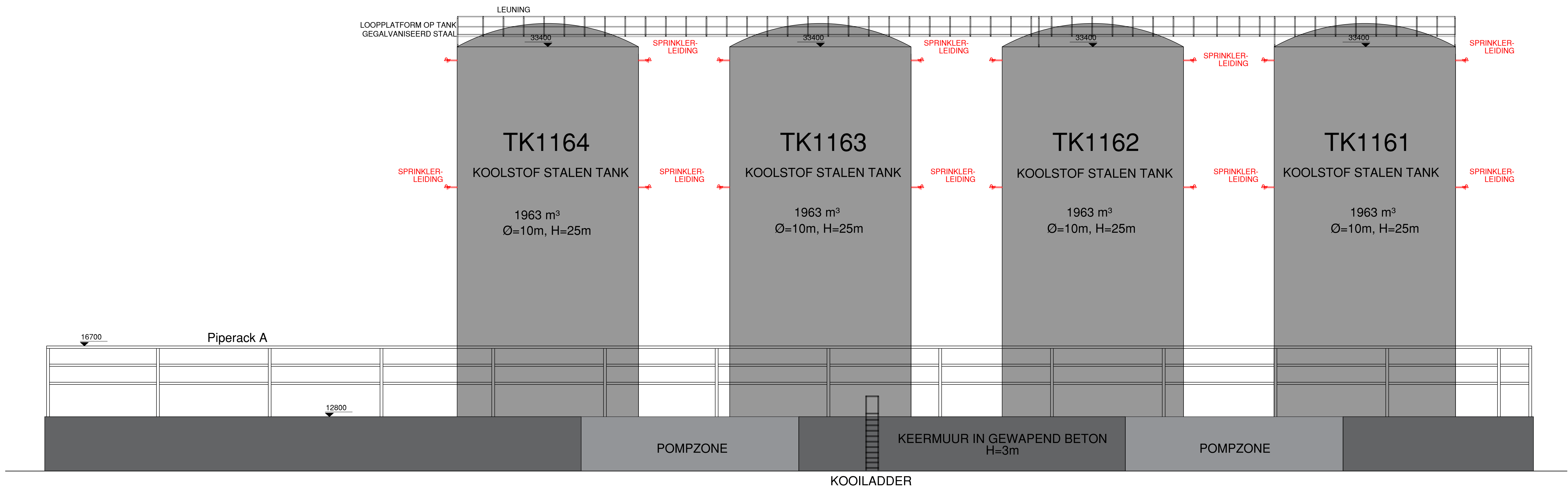
Aanzicht oost
