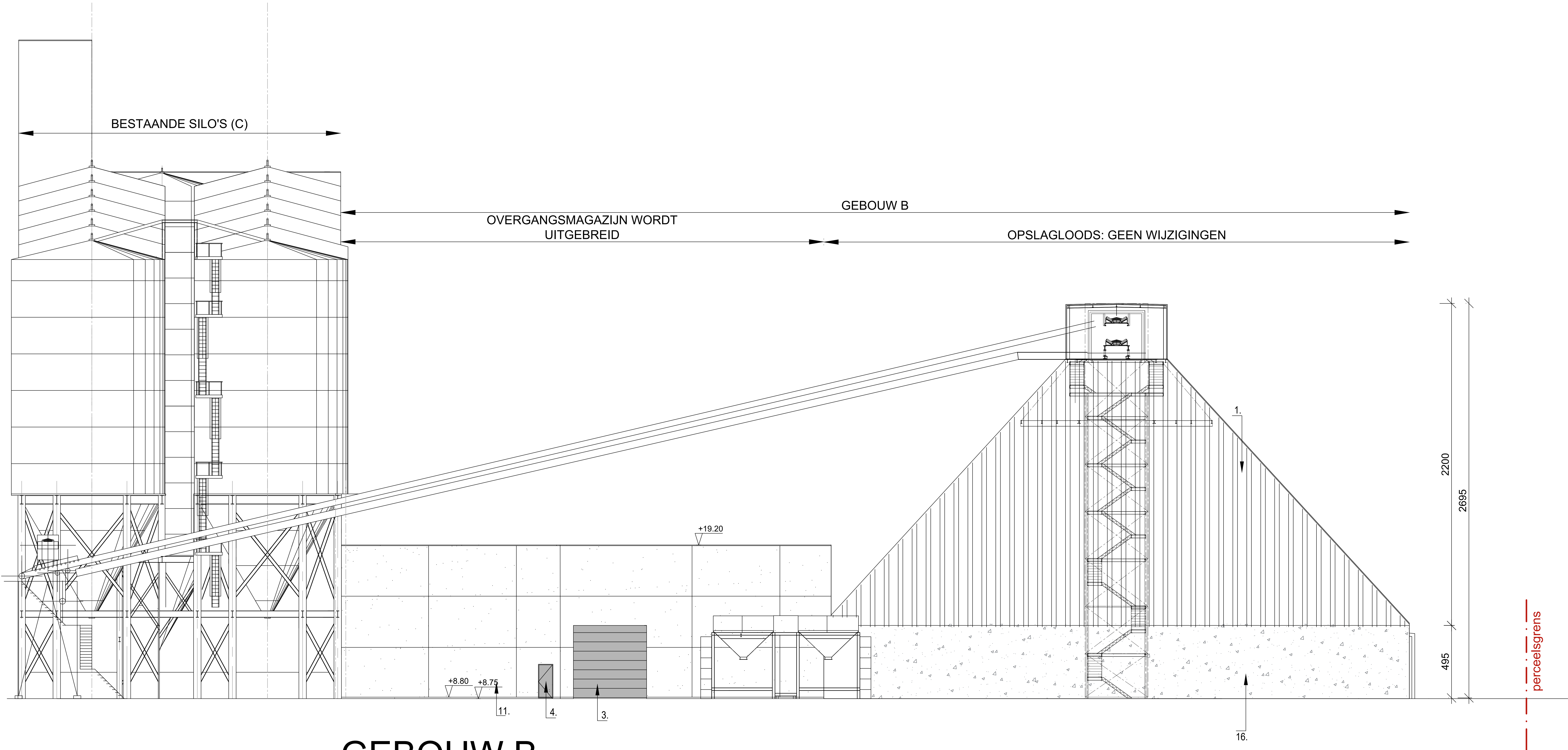
GEBOUW B GEVEL ZUID - BT = NT = VT
