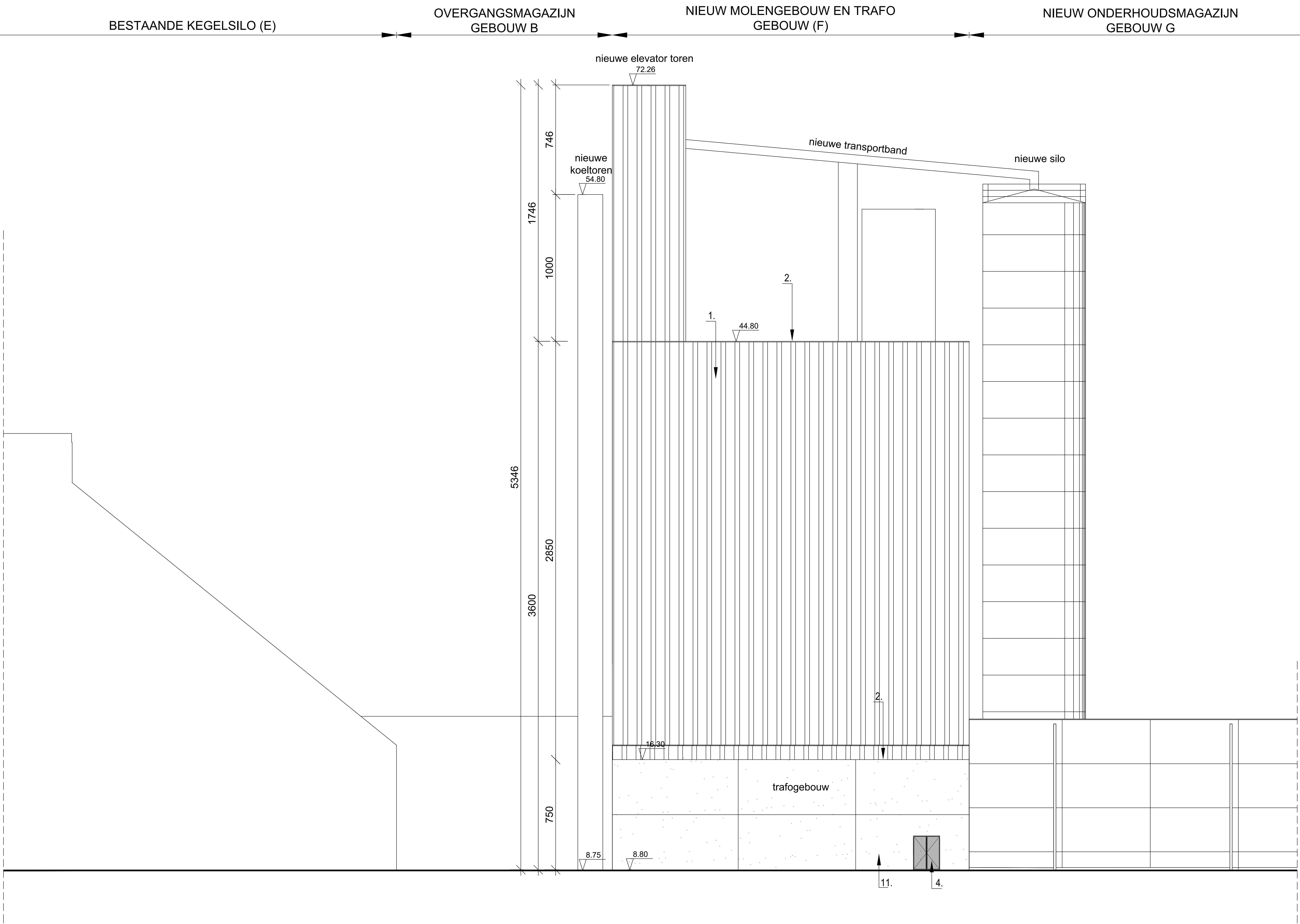
GEBOUW F - NIEUW MOLENGEBOUW GEVEL NOORD - NIEUW
