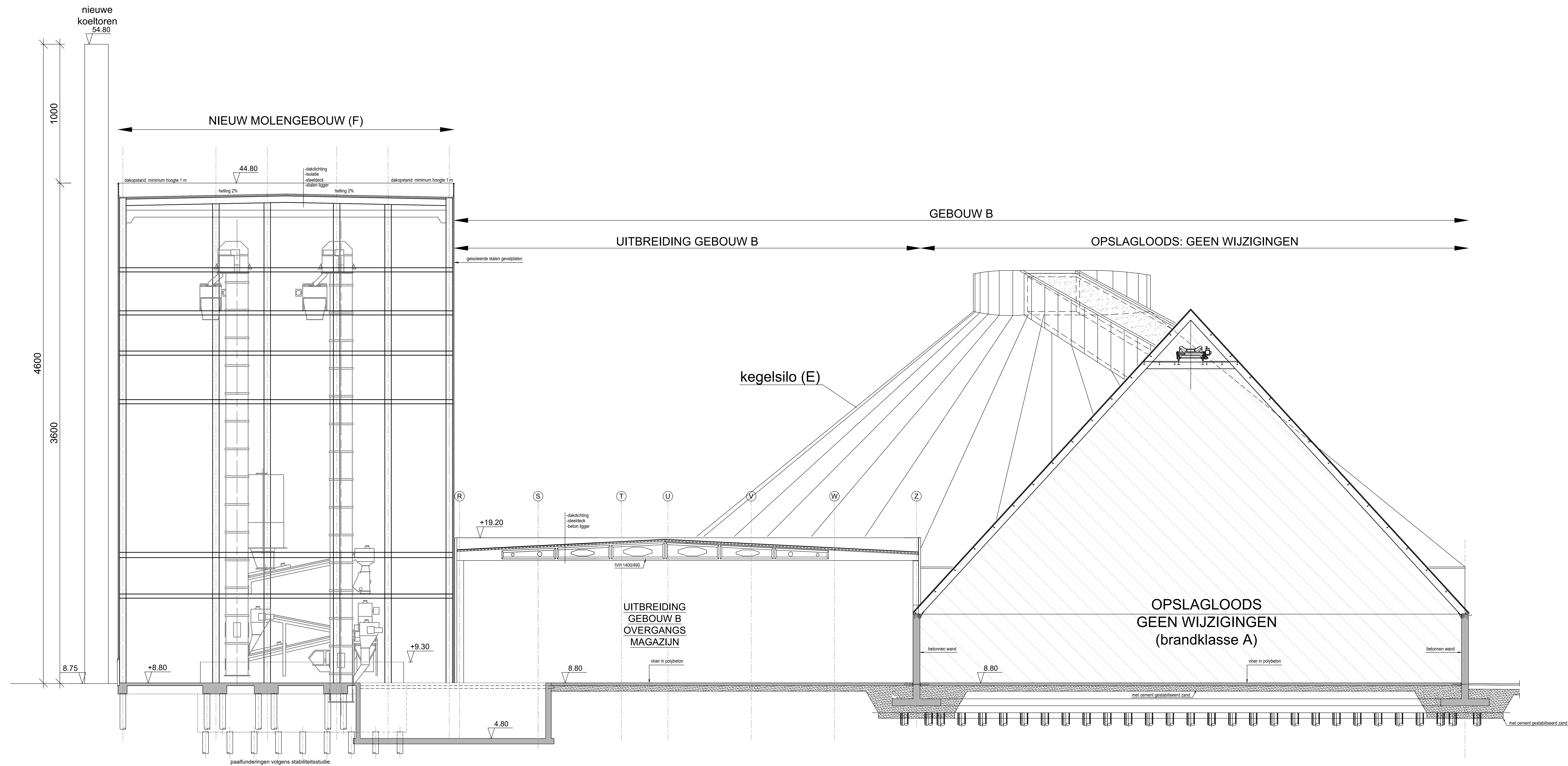
GEBOUW F - NIEUW MOLENGEBOUW SNEDE I - NIEUW
