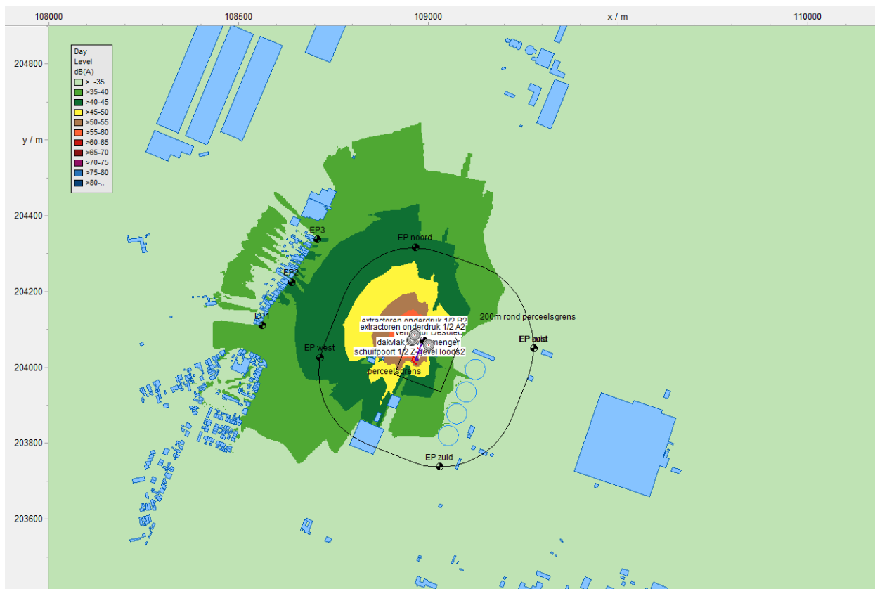
Figuur 1: Geluidscontourkaart van de geluidsbelasting van de geplande installaties met geluidsreductie bij 2 van de 4 geplande extractieventilatoren (geluidsreductie van minimaal 10 dB(A))
