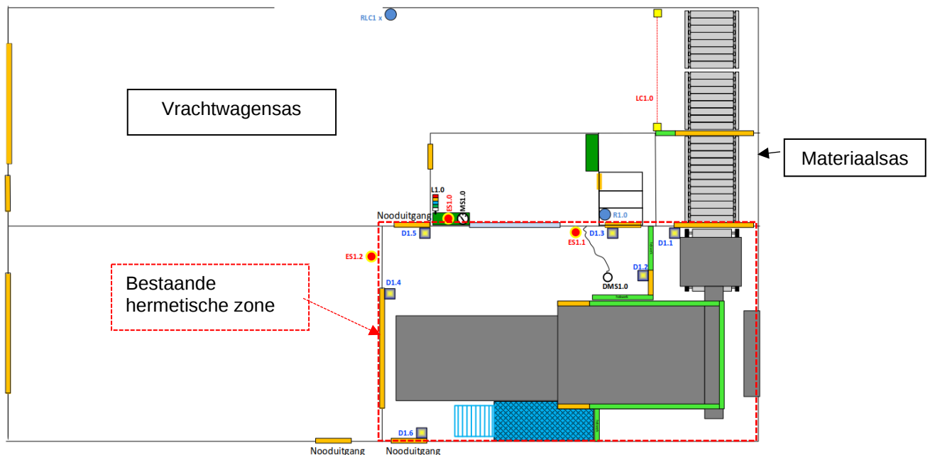
Figuur 6 Inrichting loods 2B
