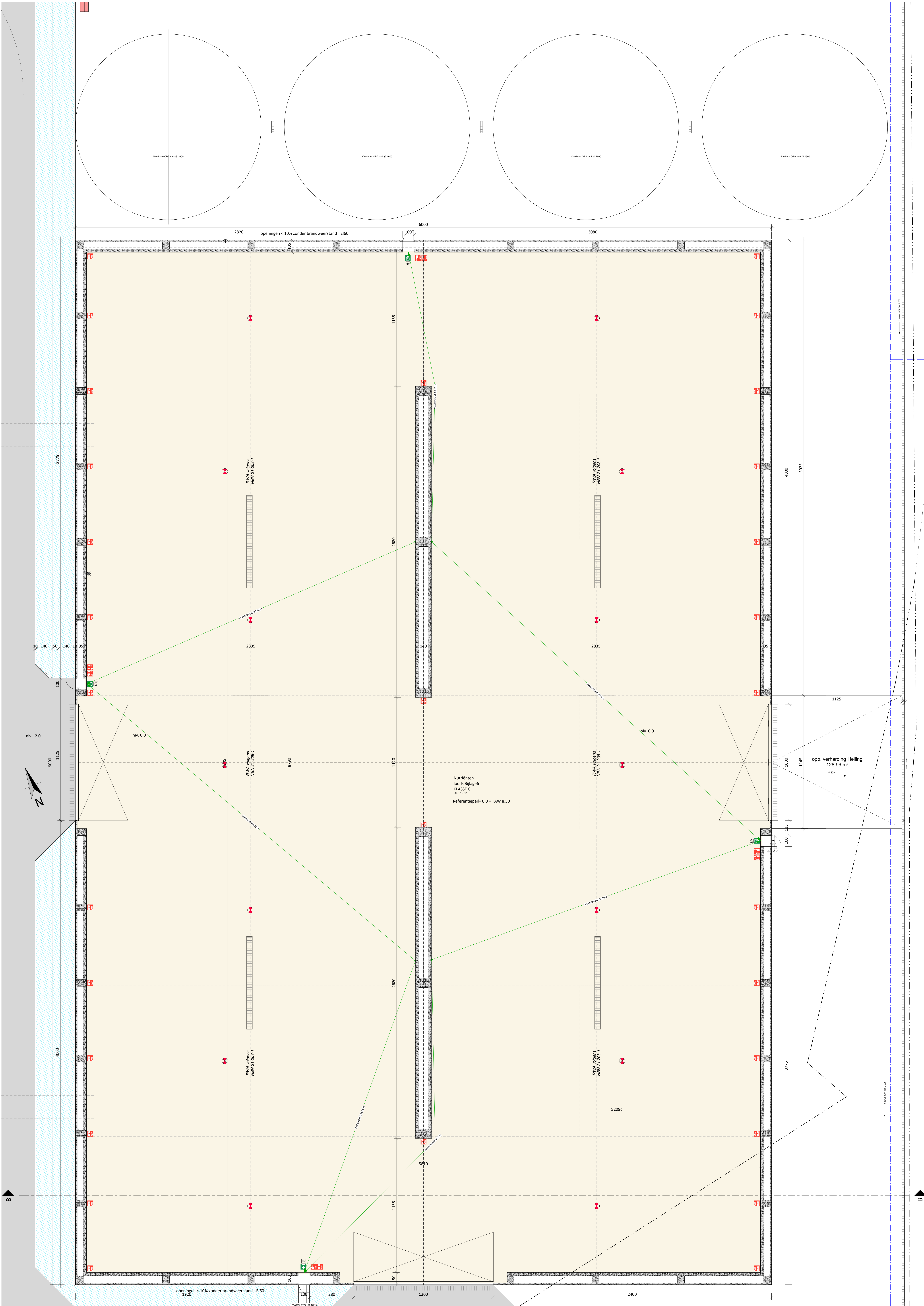
Grondplan gelijkvloers Nutriënten loods | Nieuwe toestand | 1 : 100
