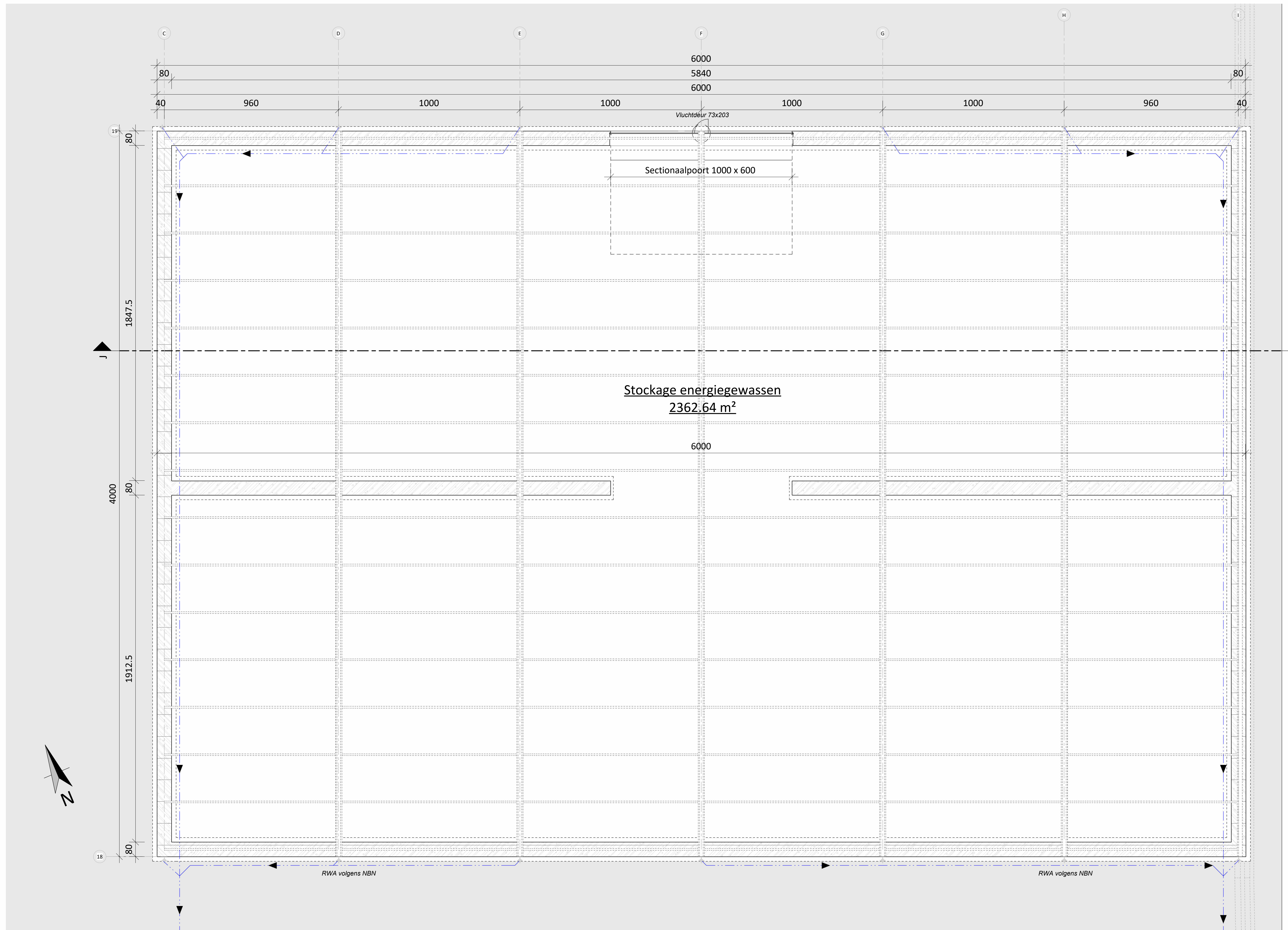
Grondplan gelijkvloers Stockage energiegewassen | Nieuwe toestand | 1 : 100
