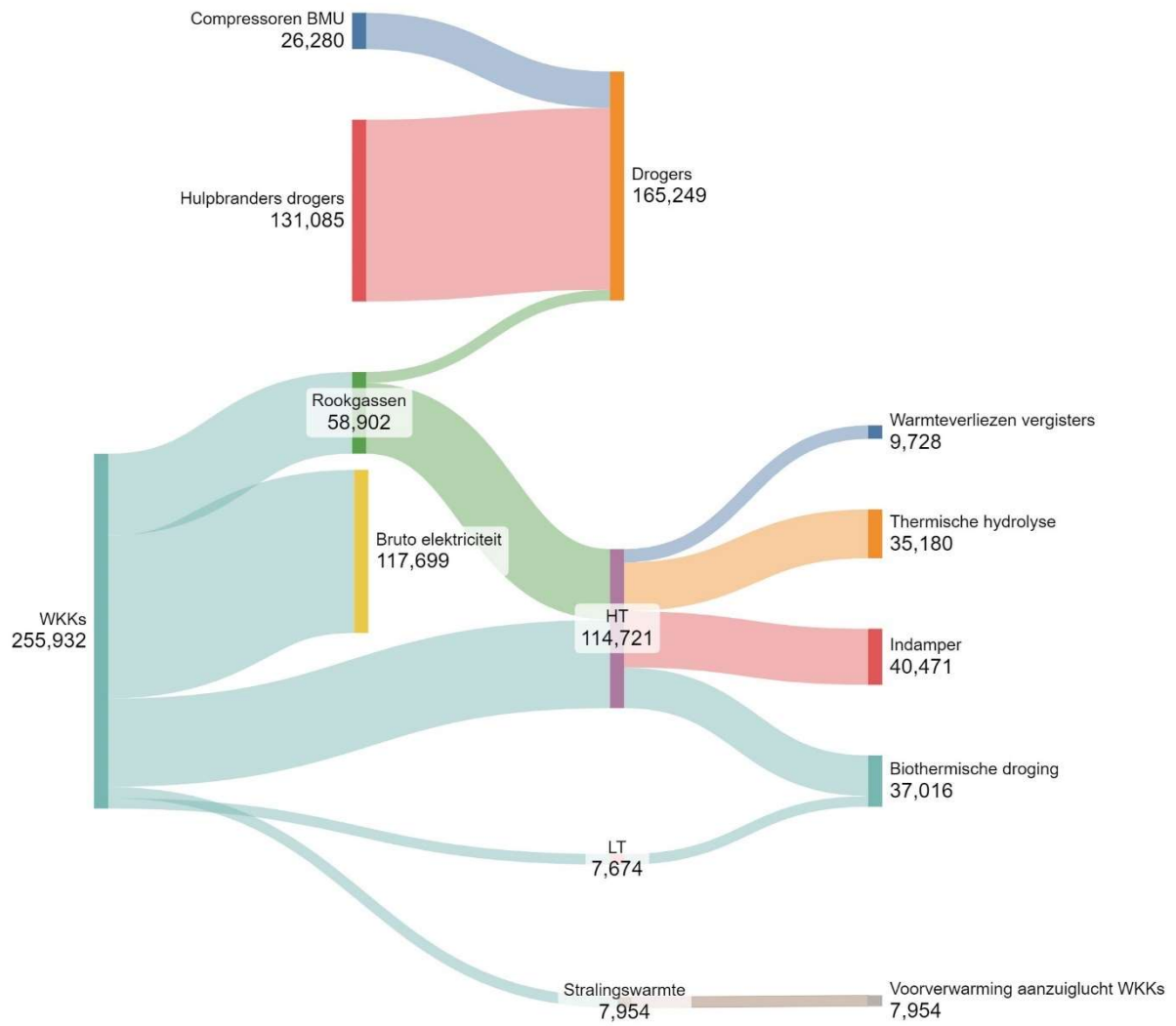
Figuur 7: Warmtestromen op jaarbasis (MWh)
