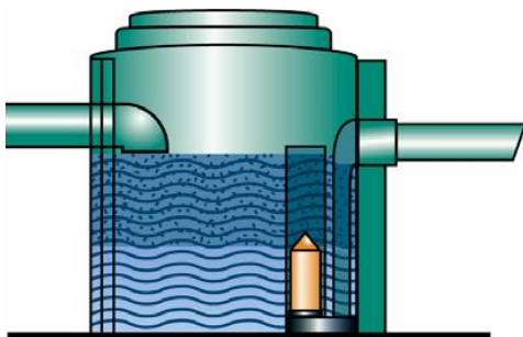
Figuur 1 KWS-scheider
