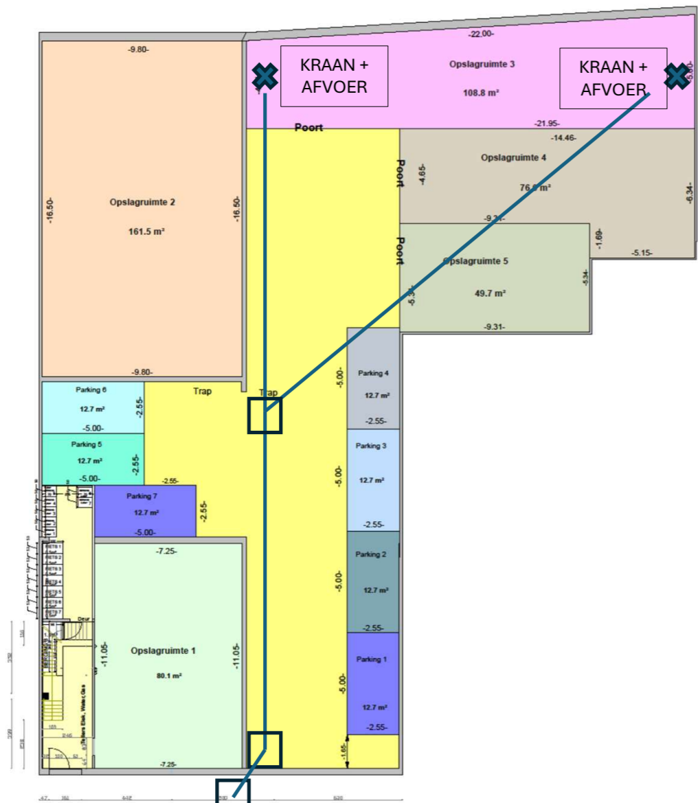
GELIJKVLOERS VAN DEN HECKESTRAAT RIOLERING
