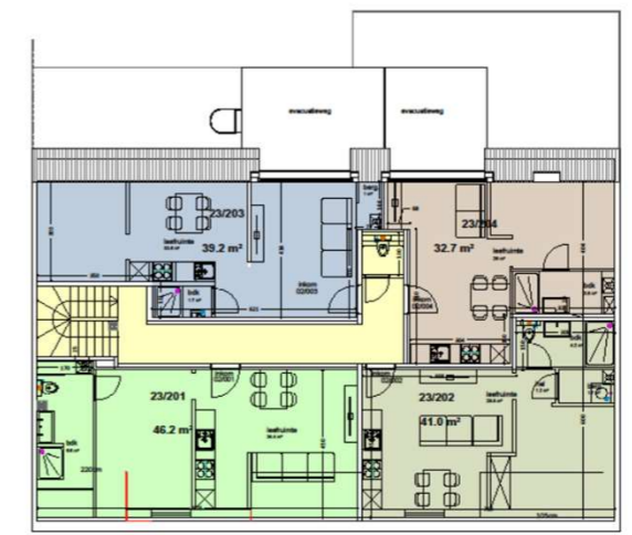
NIVEAU 02 VAN DEN HECKESTRAAT
