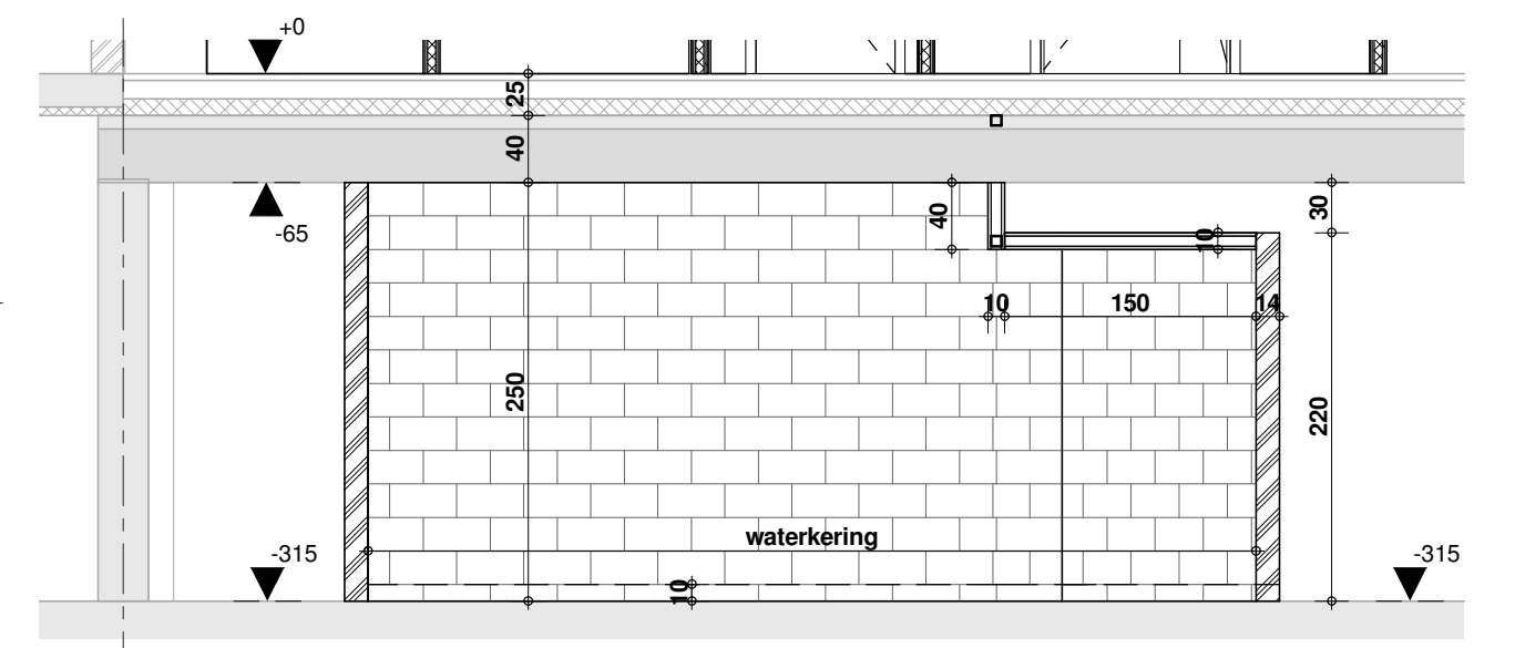
Doorsnede Y 1/50
