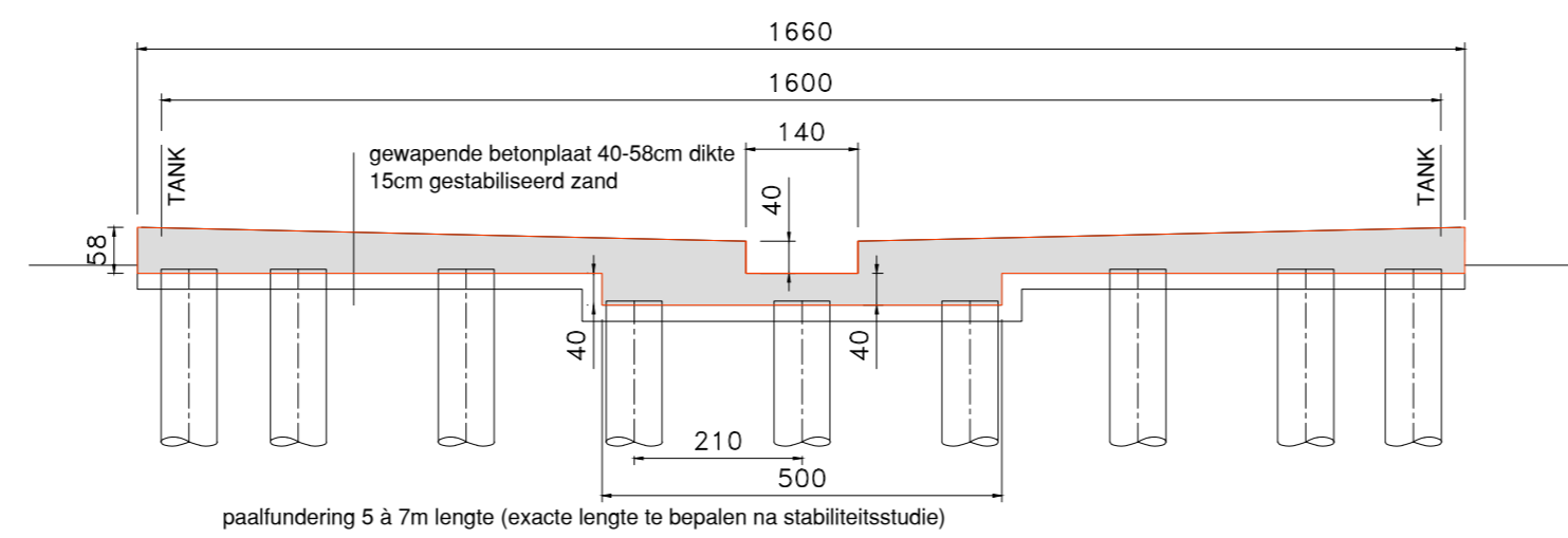
SNEDE A-A
