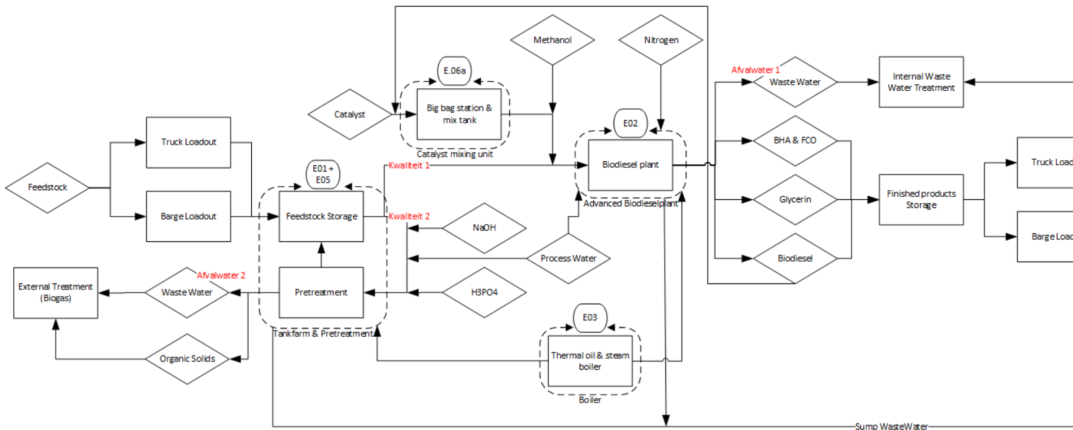
Figuur 1 Processchema nieuwe advanced biodieselplant
