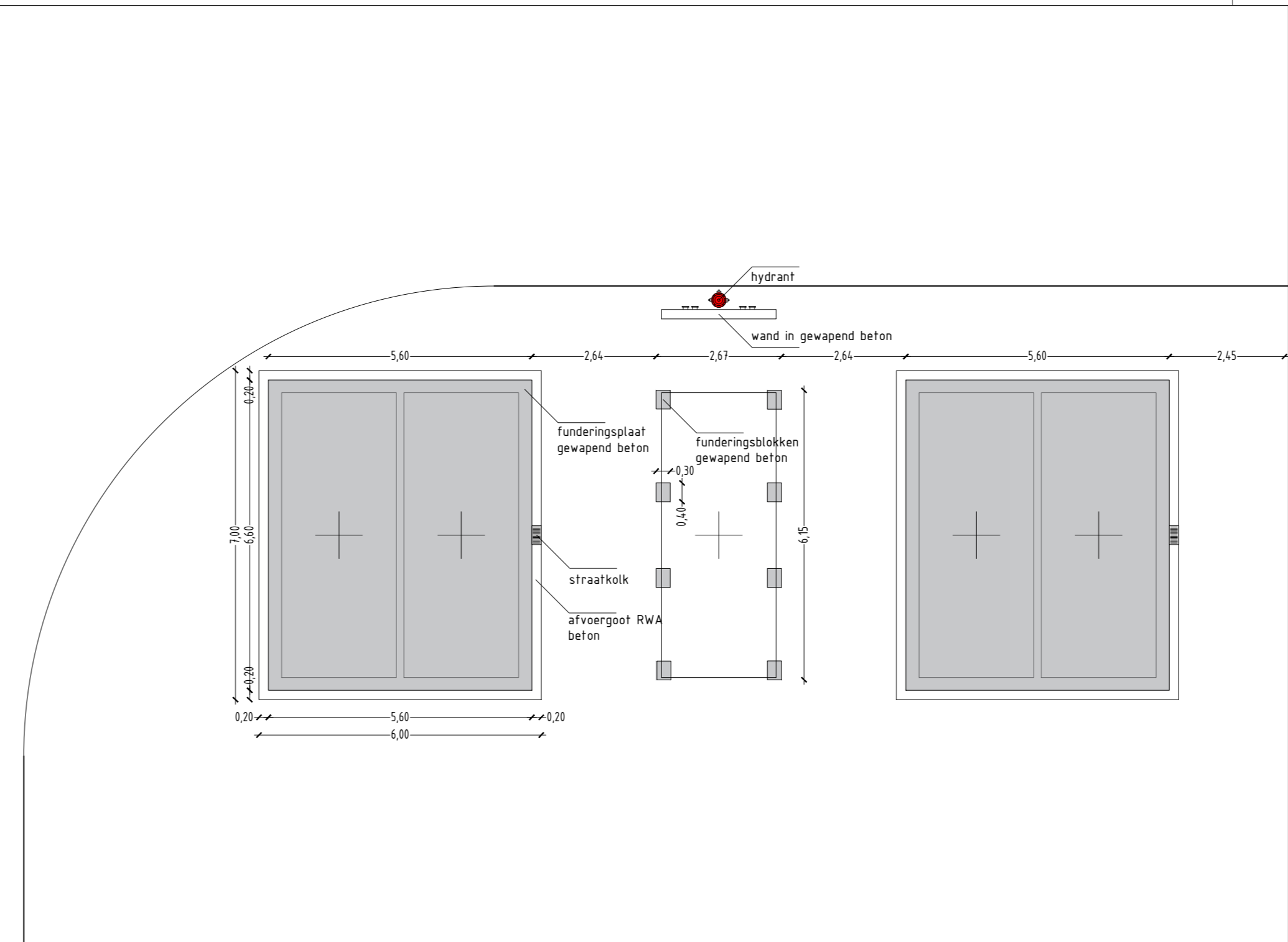
BESS - Plan gelijkvloers nieuwe toestand
