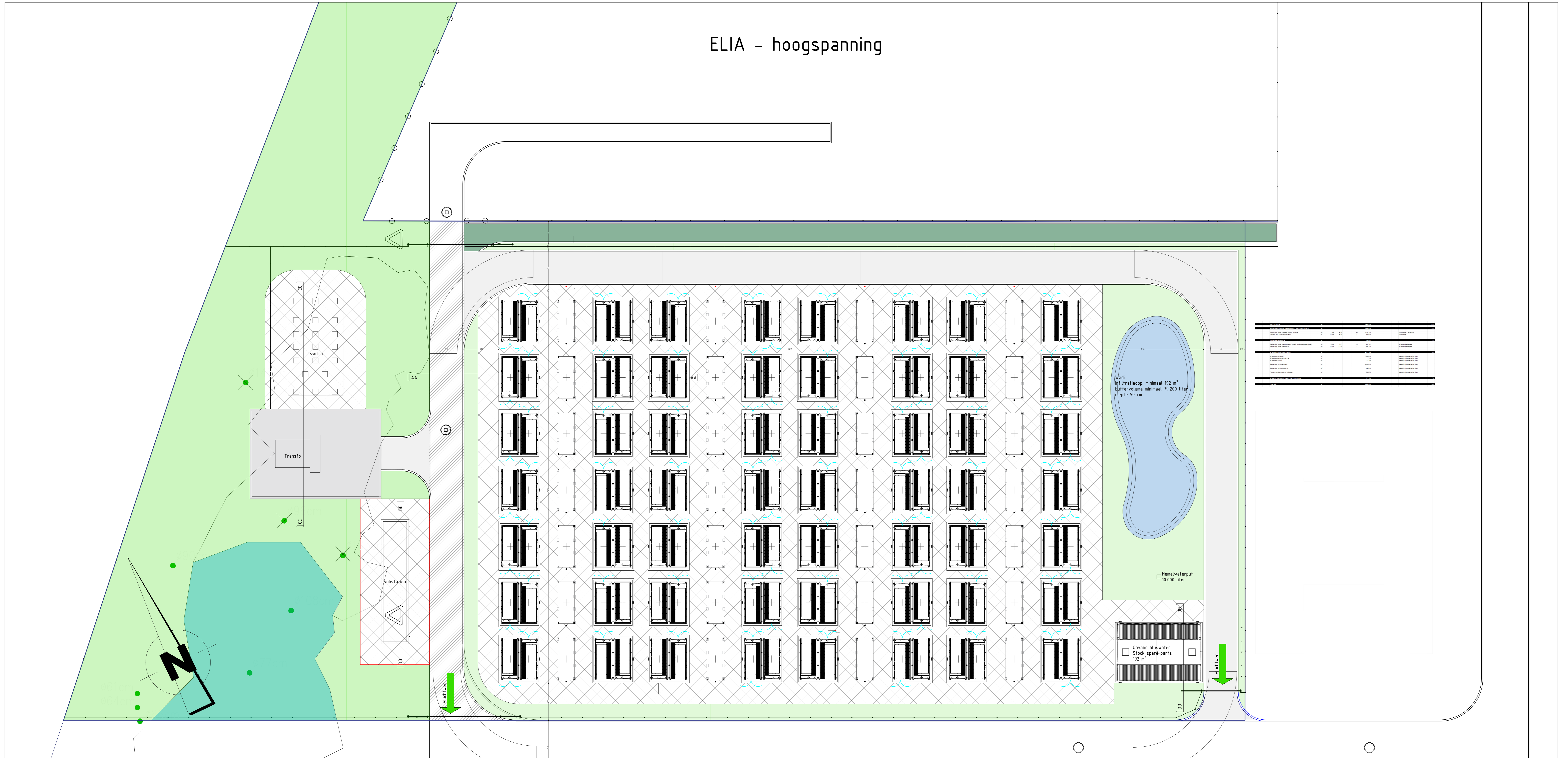
BESS - Plan gelijkvloers nieuwe toestand
