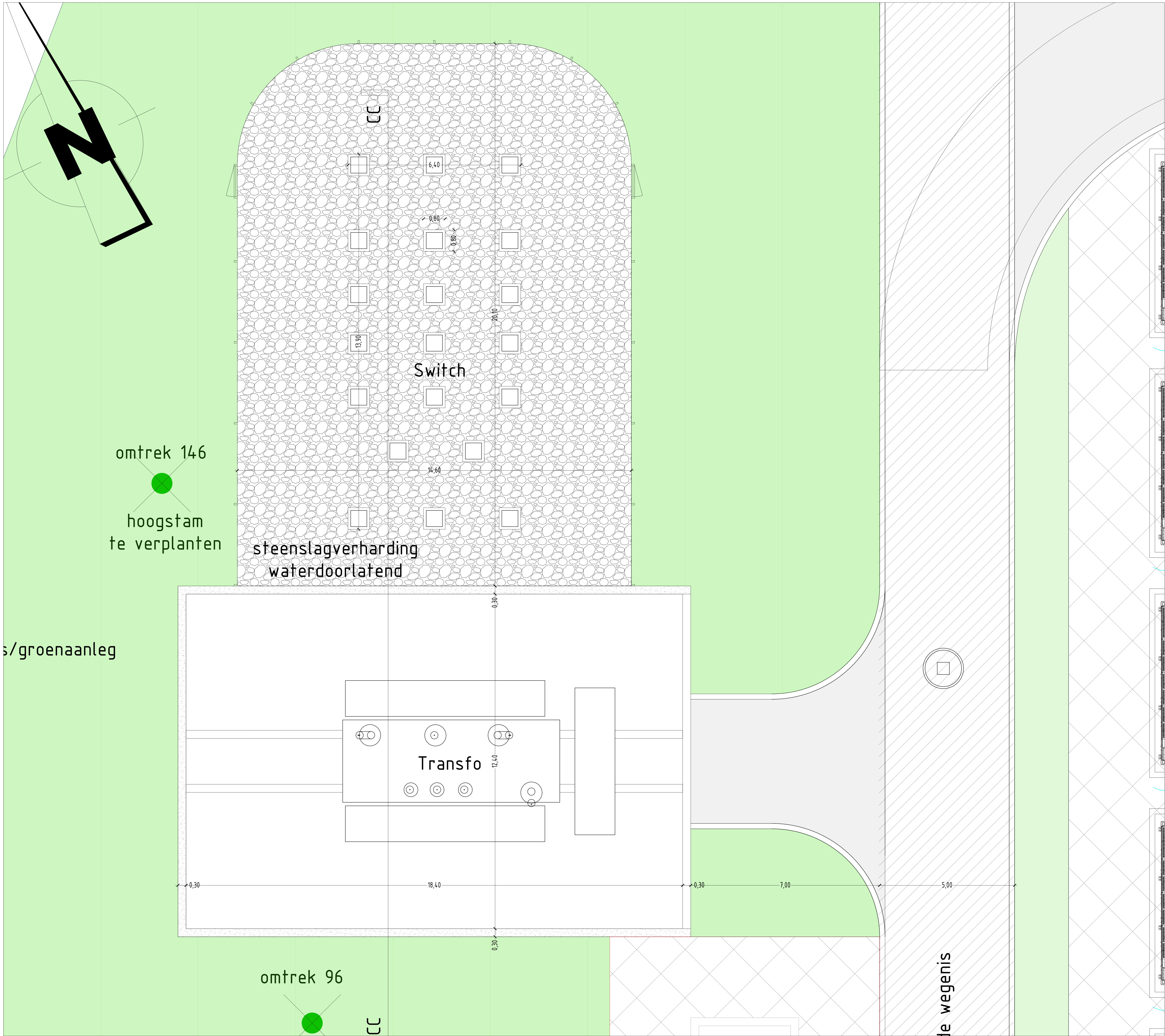
Plan +0 - Transfo HV & Switch
