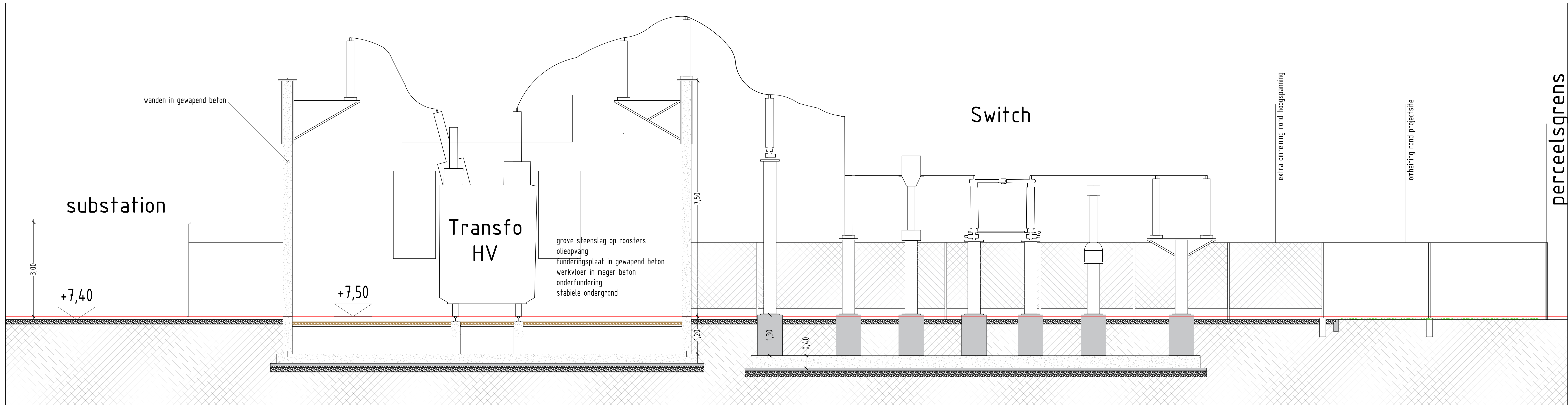
Snede CC - Transfo HV & Switch
