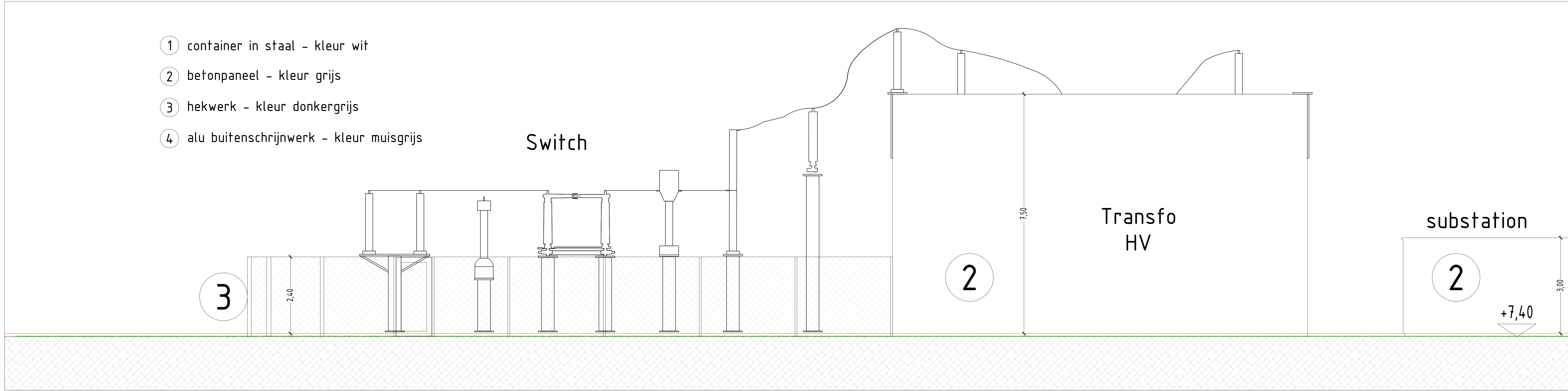
Gevel West - Transfo HV & Switch
