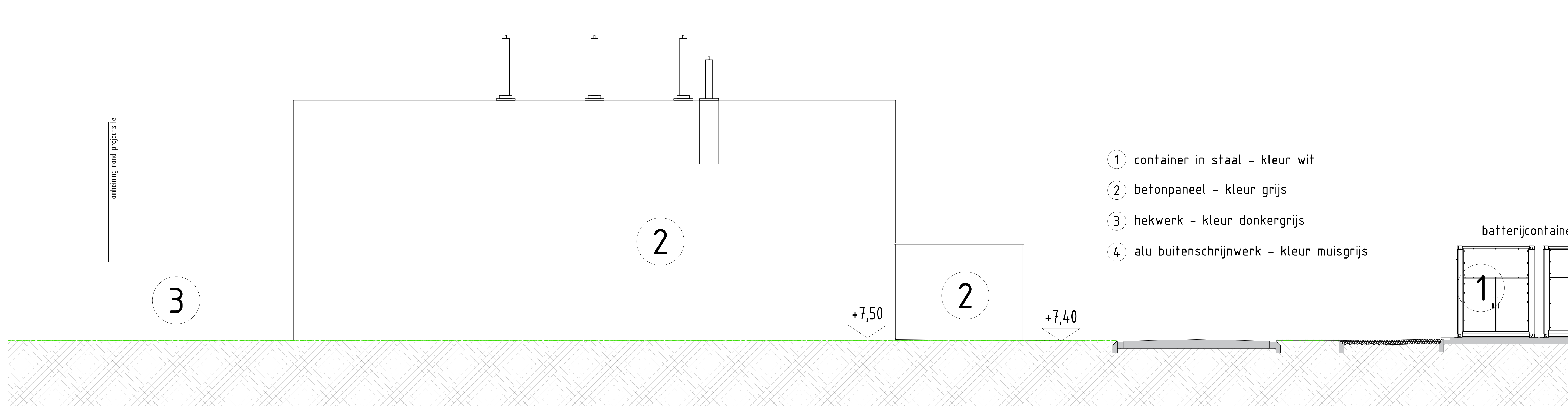
Gevel Zuid - Transfo HV & Switch
