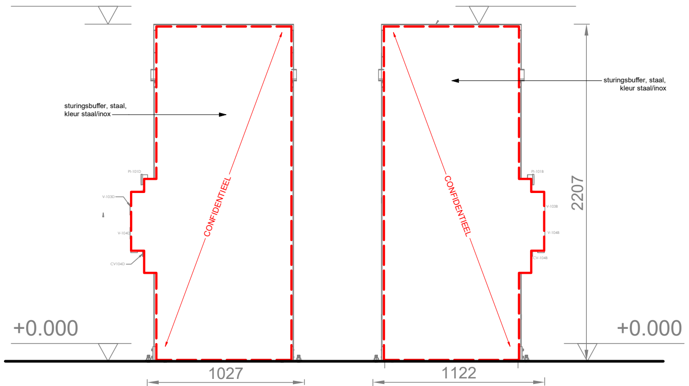
AANZICHT OOST
