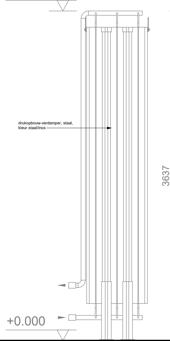
AANZICHT OOST
