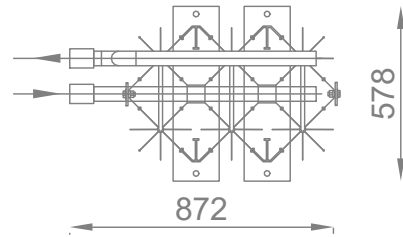
GRONDPLAN DRUKOPBOU-VERDAMPER
