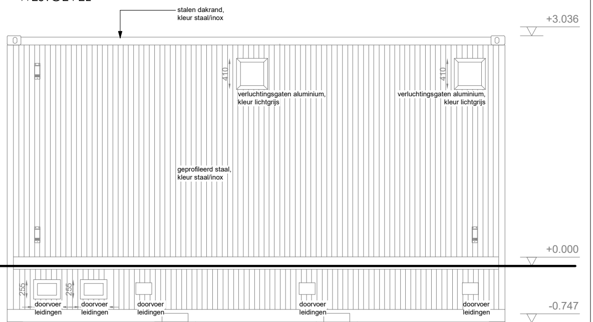
OOSTGEVEL
