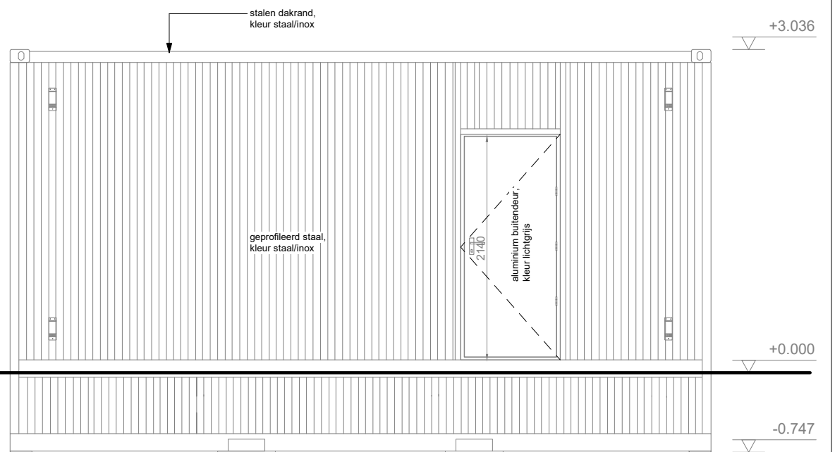
WESTGEVEL
