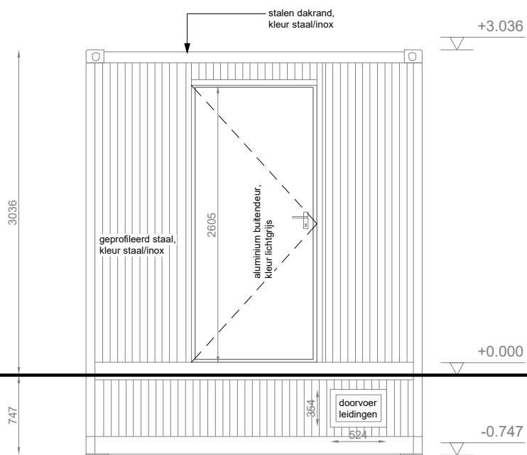
NOORDGEVEL
