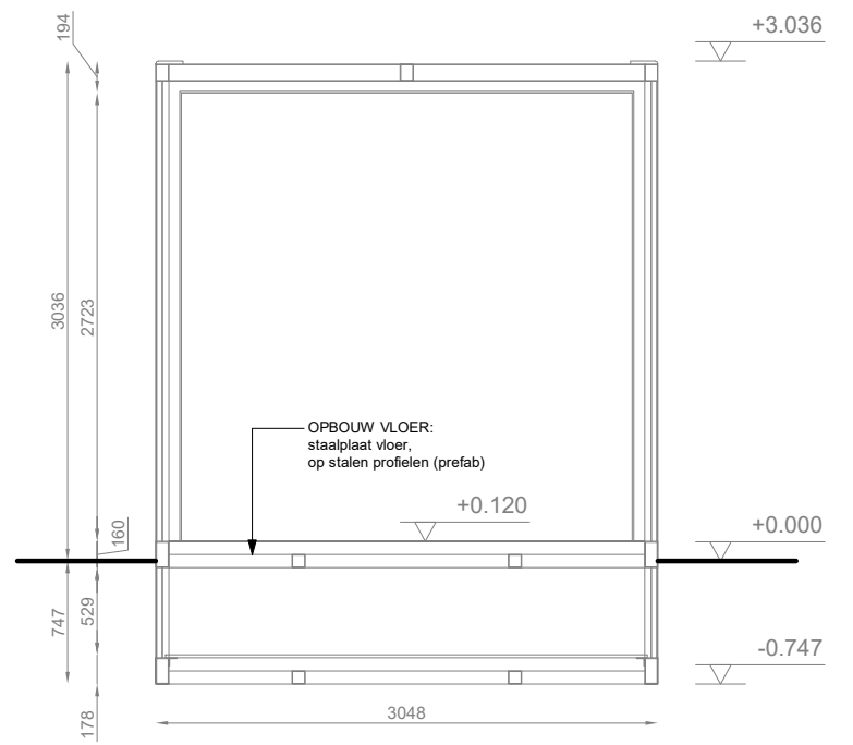
SNEDE A
