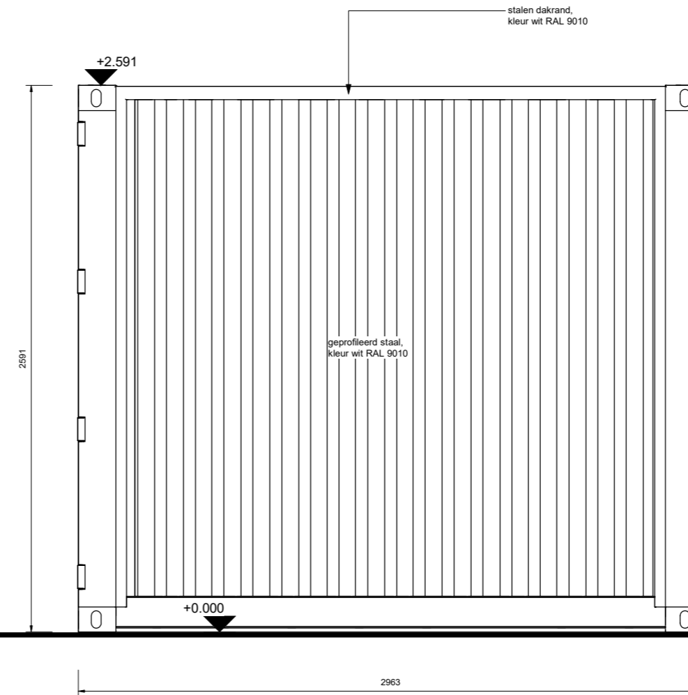
3 Zuidgevel technisch lokaal 1 : 25
