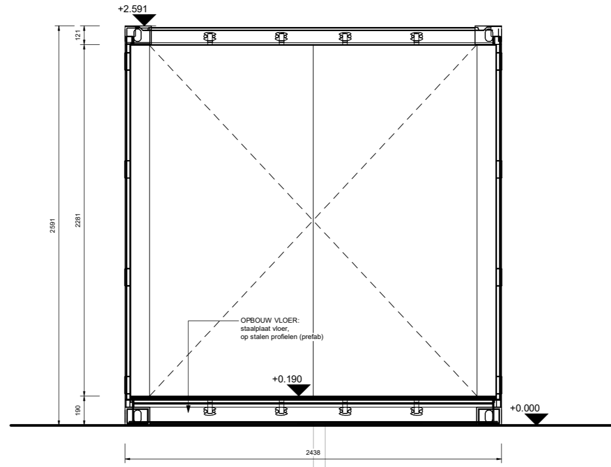
6 Snede technisch lokaal 1 : 25
