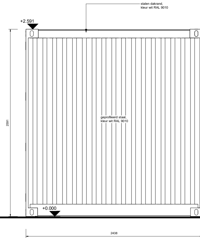
5 Oostgevel technisch lokaal 1 : 25
