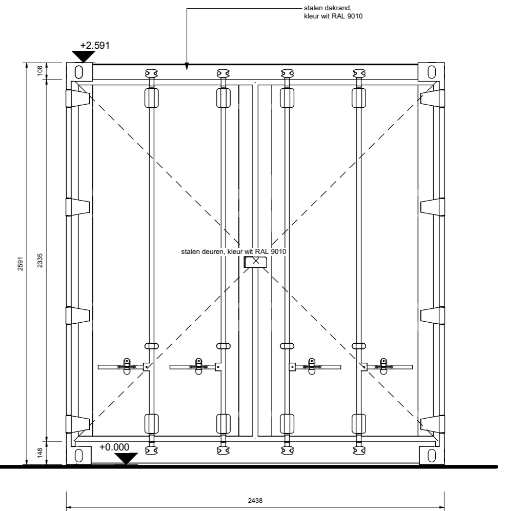
2 Westgevel technisch lokaal 1 : 25
