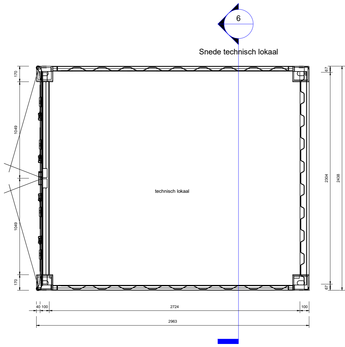
1 Grondplan technisch lokaal 1 : 25
