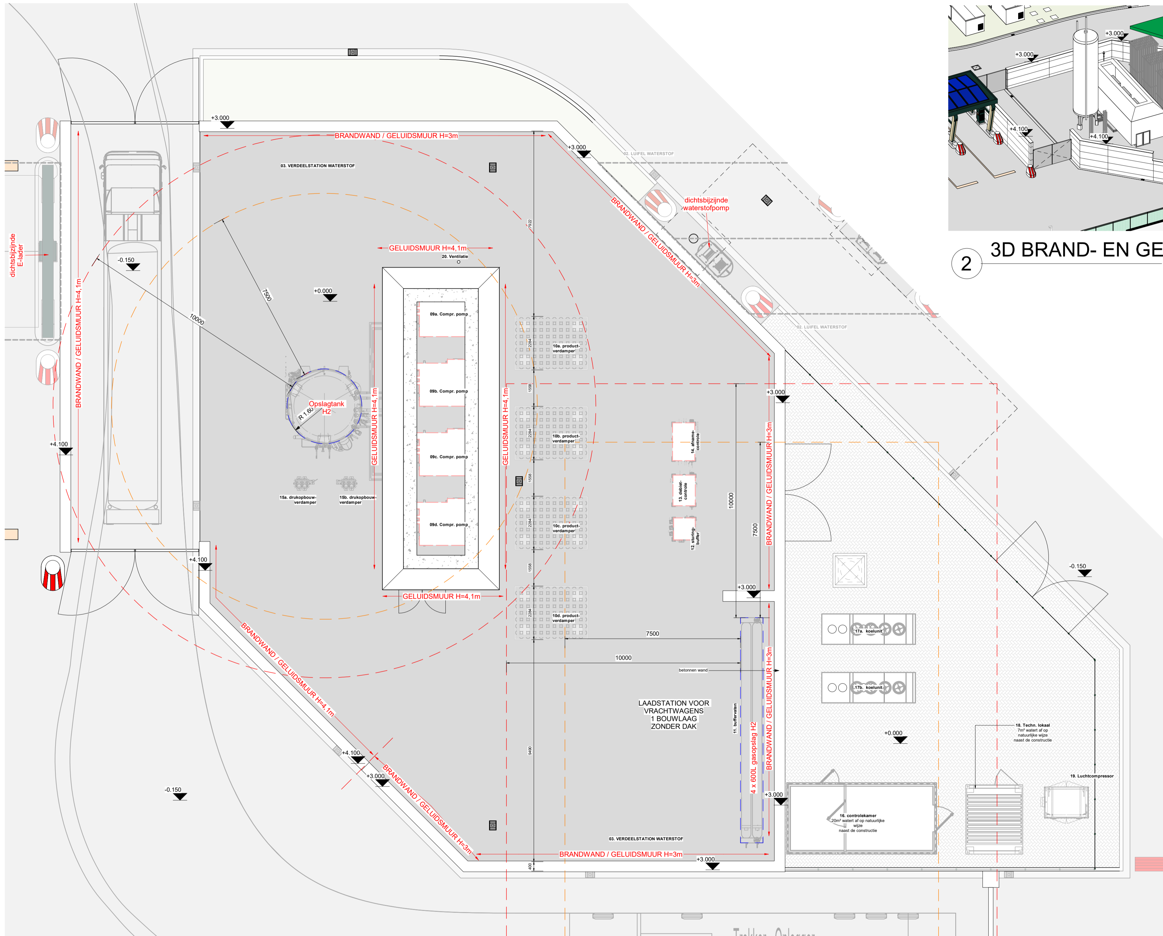
1 Brand- en geluidsmuren - veiligheidsafstanden 1 : 100
