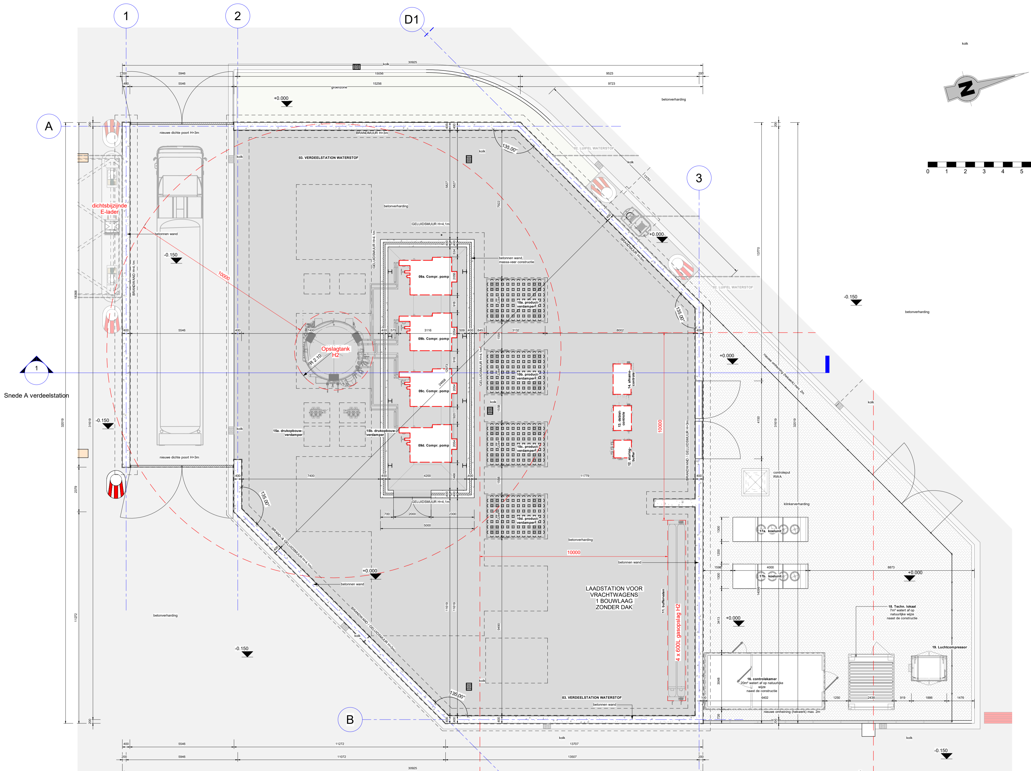
1 gelijkvloers verdeelstation waterstof 1 : 100
