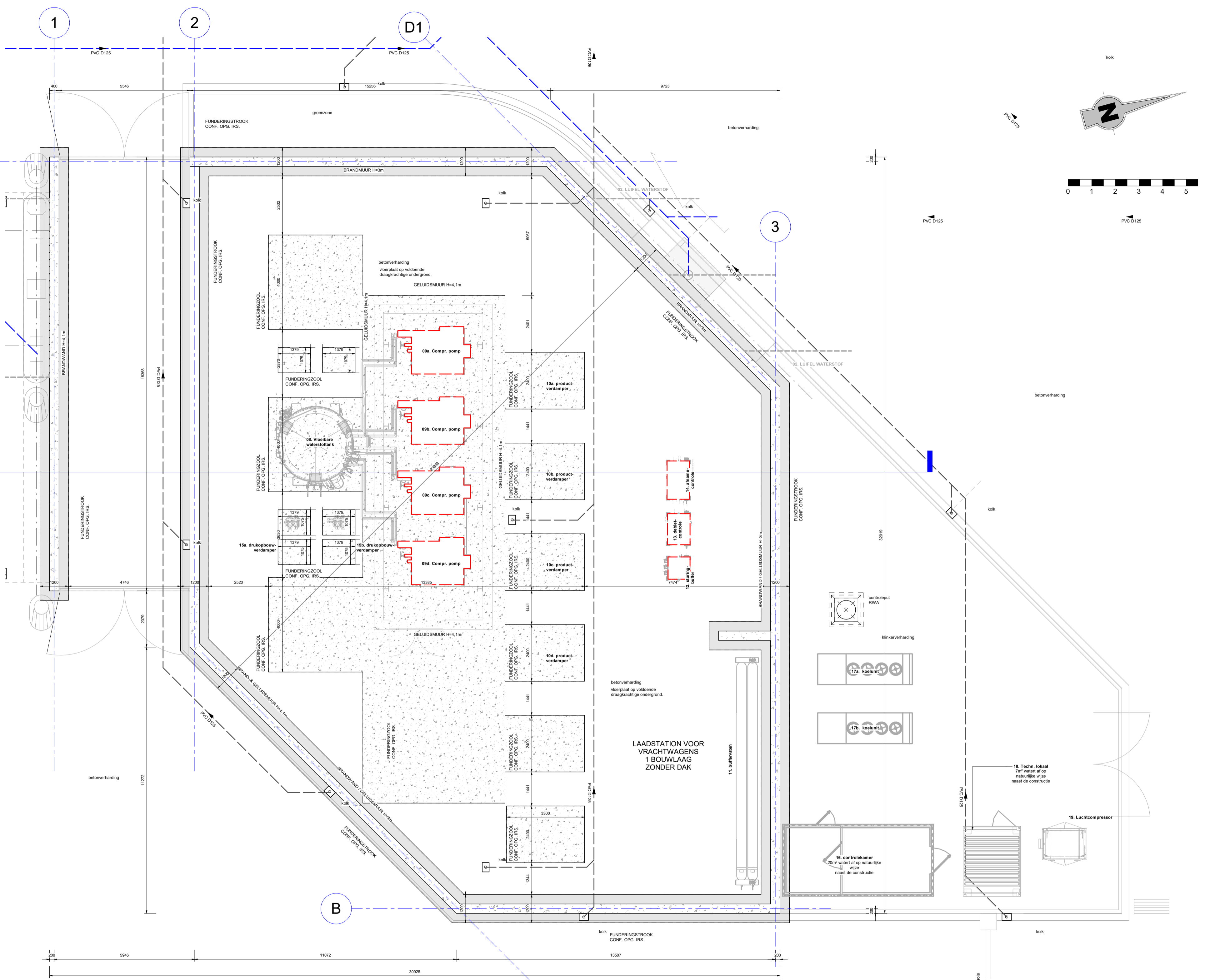
1 Fundering verdeelstation waterstof 1 : 100
