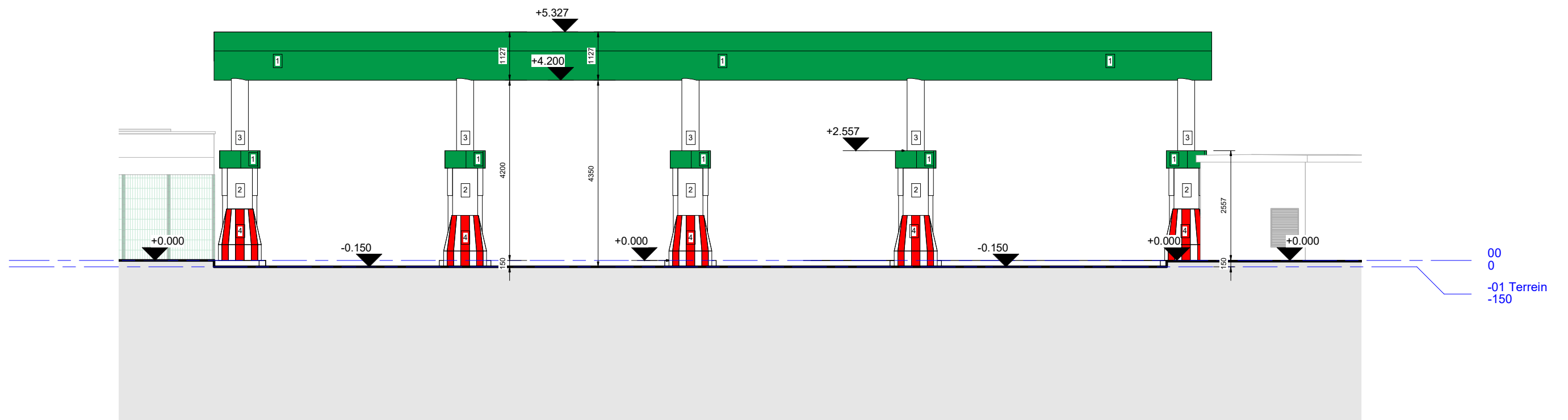
1 Oostgevel luifel waterstof 1 : 100
