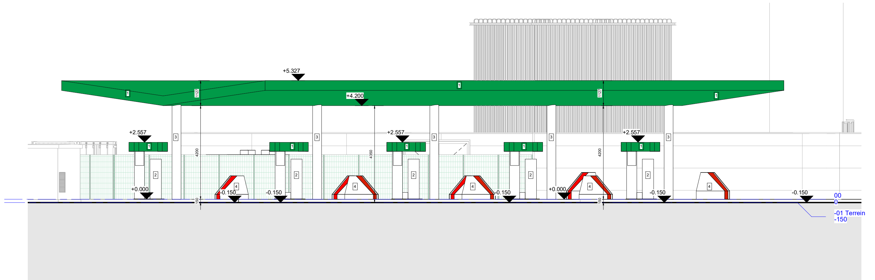
1 Noordgevel luifel waterstof 1 : 100
