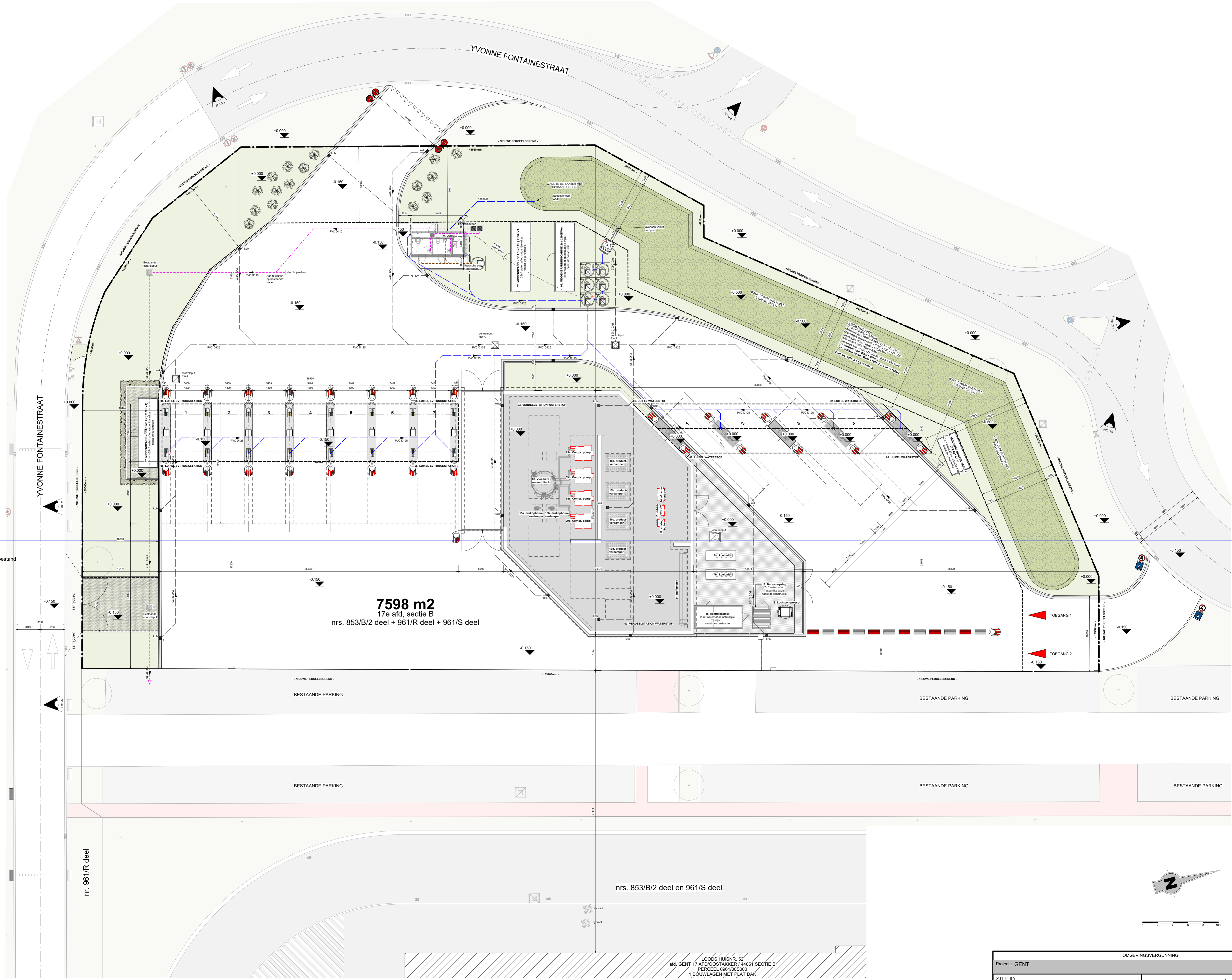
1 Inplanting totaal - Nieuwe toestand riolering 1 : 200
