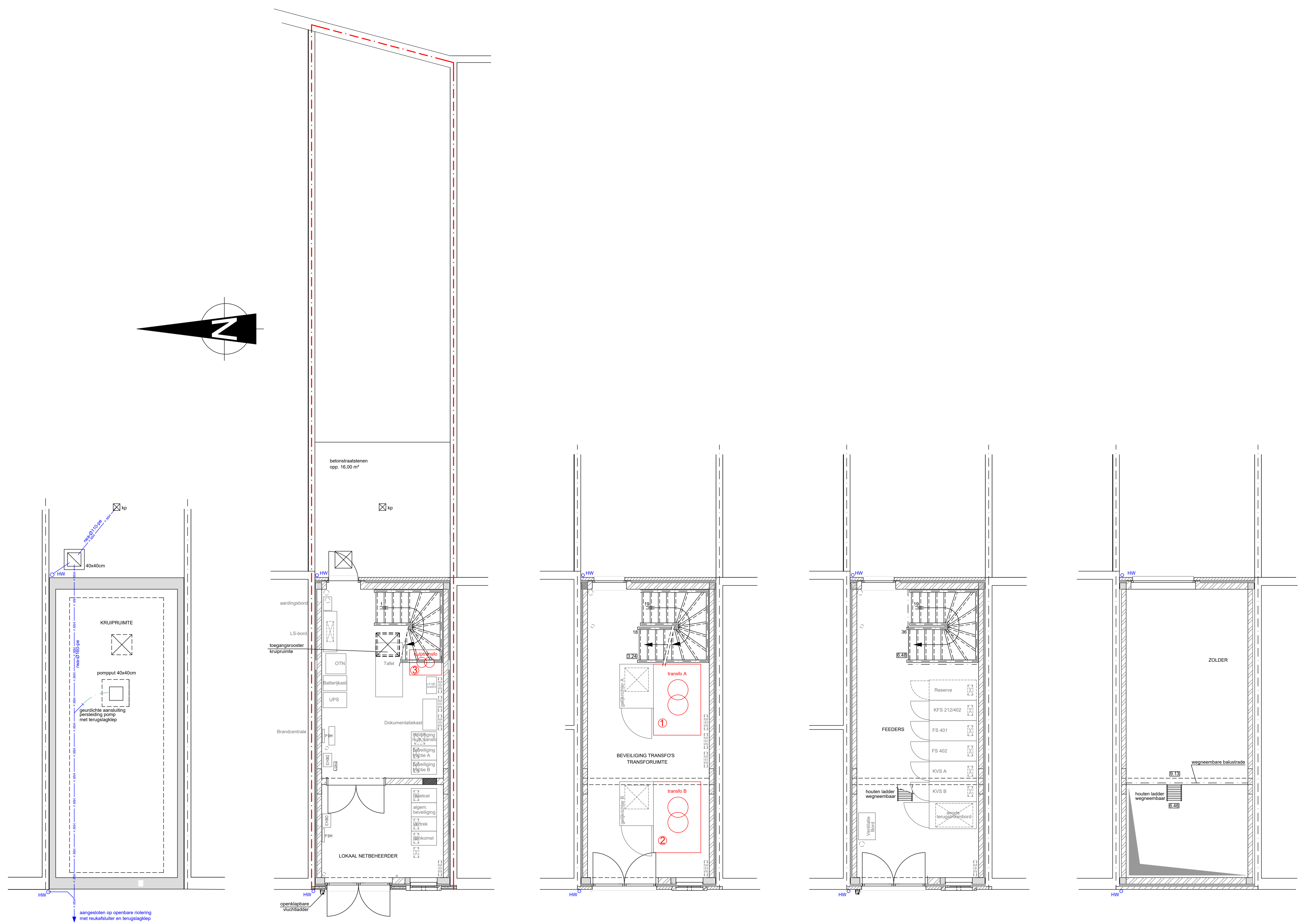
KRUIPRUIMTE (-1.40)
