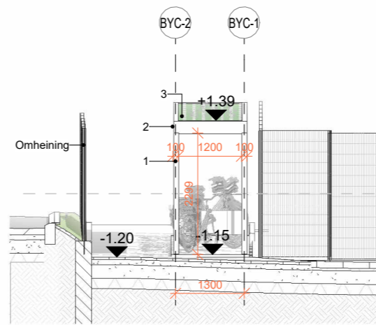
ZUIDGEVEL SCHAAL 1:100
