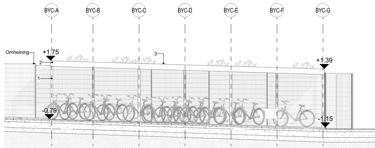
WESTGEVEL SCHAAL 1:100
