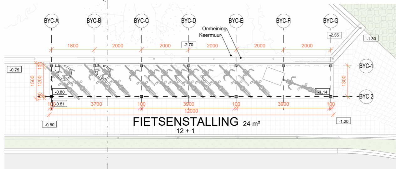
GELIJKVLOERS SCHAAL 1:100
