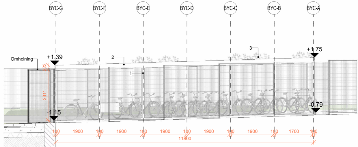
OOSTGEVEL SCHAAL 1:100
