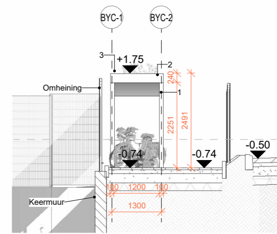
NOORDGEVEL SCHAAL 1:100
