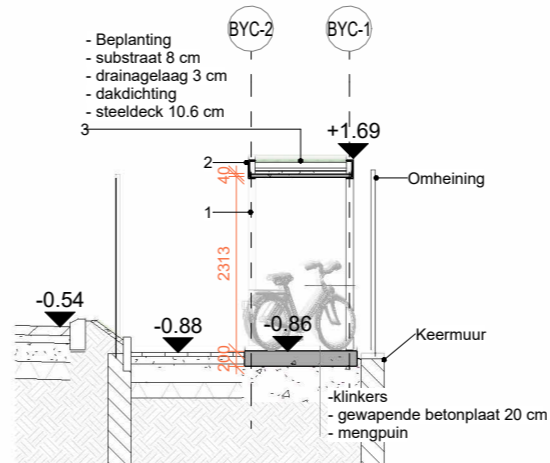
SNEDE G-G' SCHAAL 1:100
