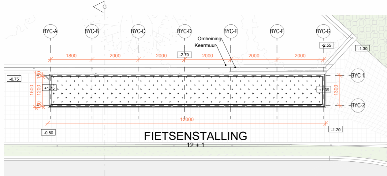
DAKPLAN SCHAAL 1:100
