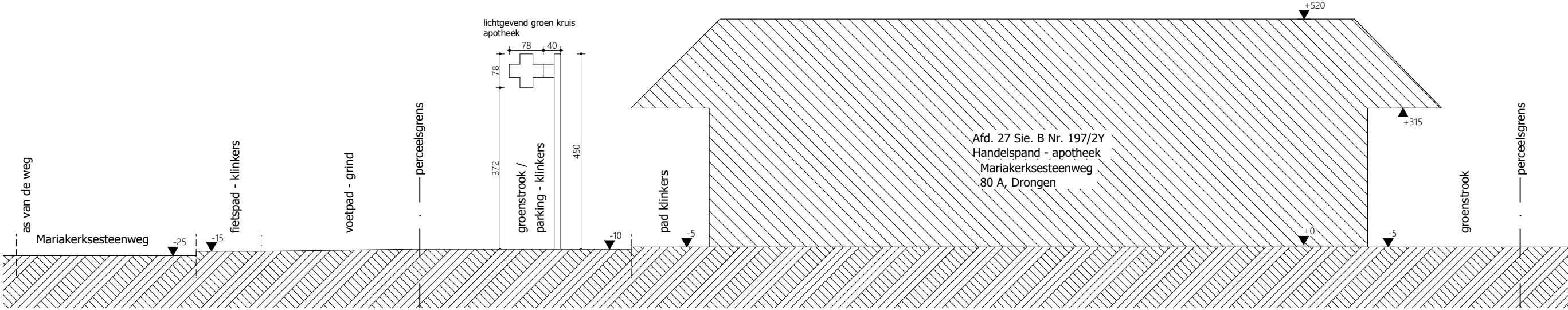
TP Terreinprofiel B - vergunde toestand 1:100
