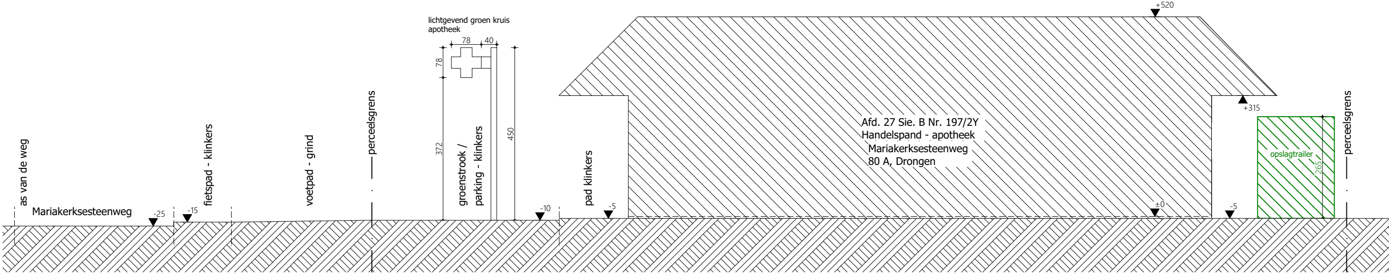
TPB Terreinprofiel B - bestaande toestand 1:100
