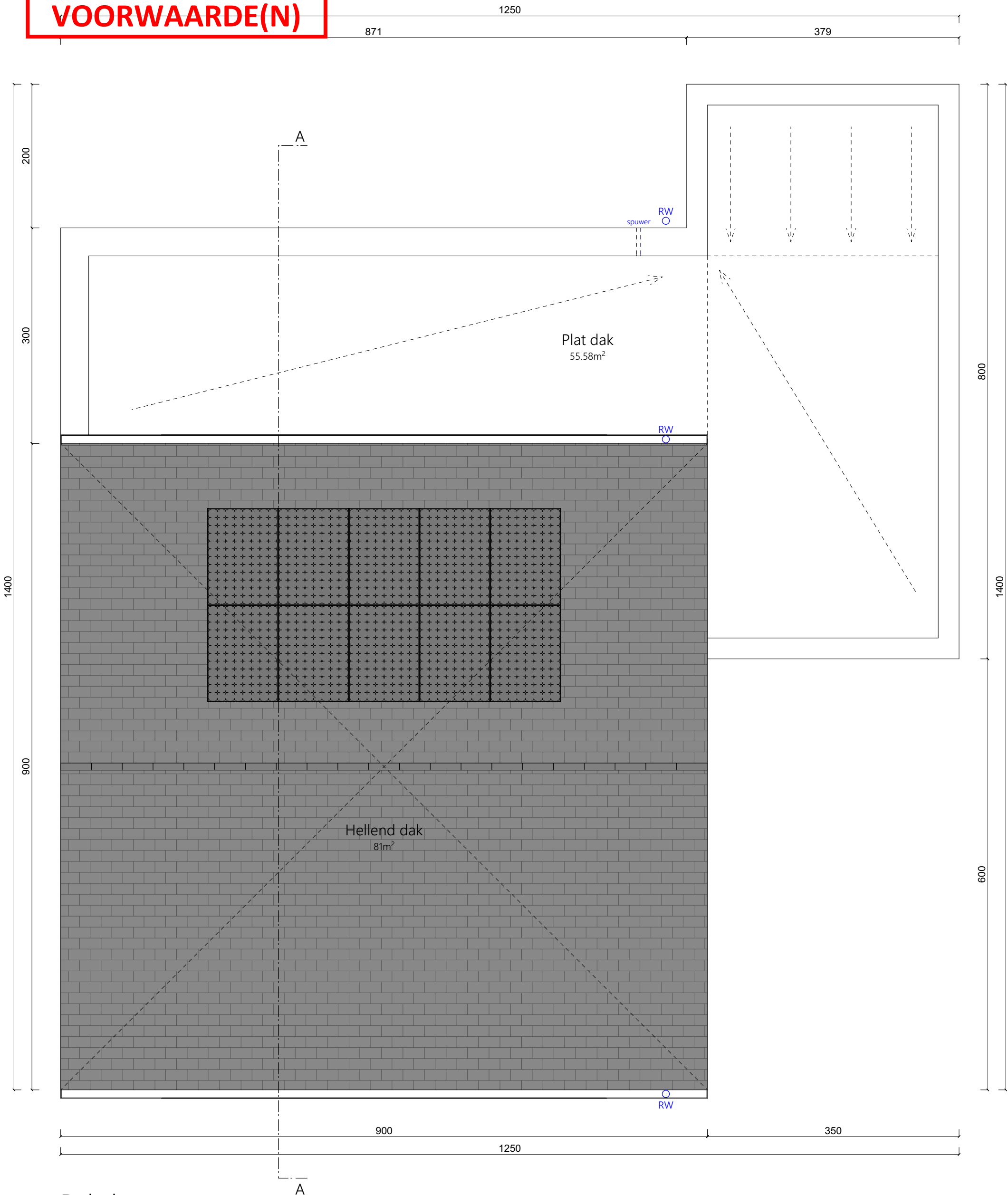
Dakplan Nieuwe toestand
