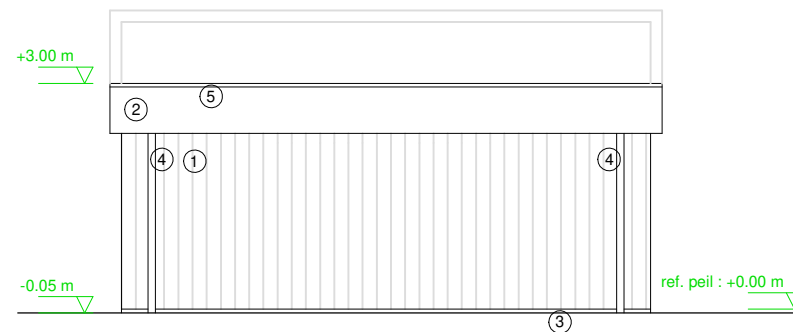
ACHTERGEVEL bijgebouw
