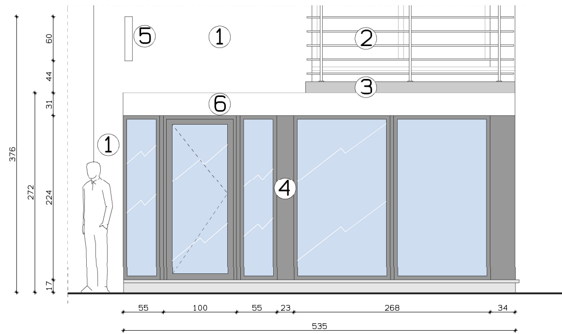
BESTAANDE TOESTAND VOORGEVEL
