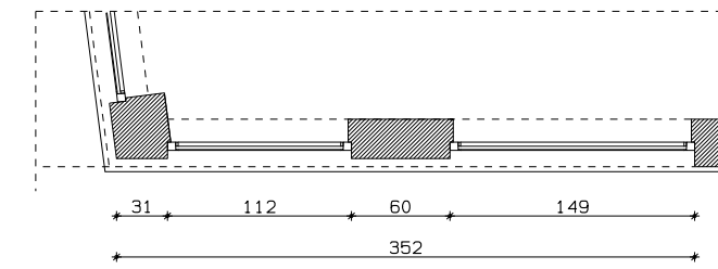
GRONDPLAN ZIJGEVEL
