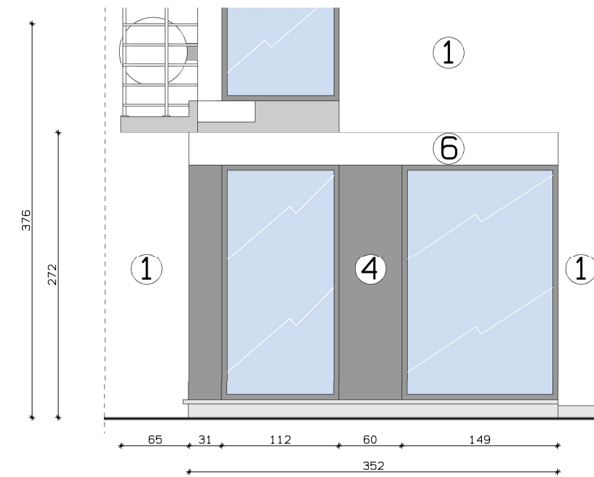
BESTAANDE TOESTAND ZIJGEVEL
