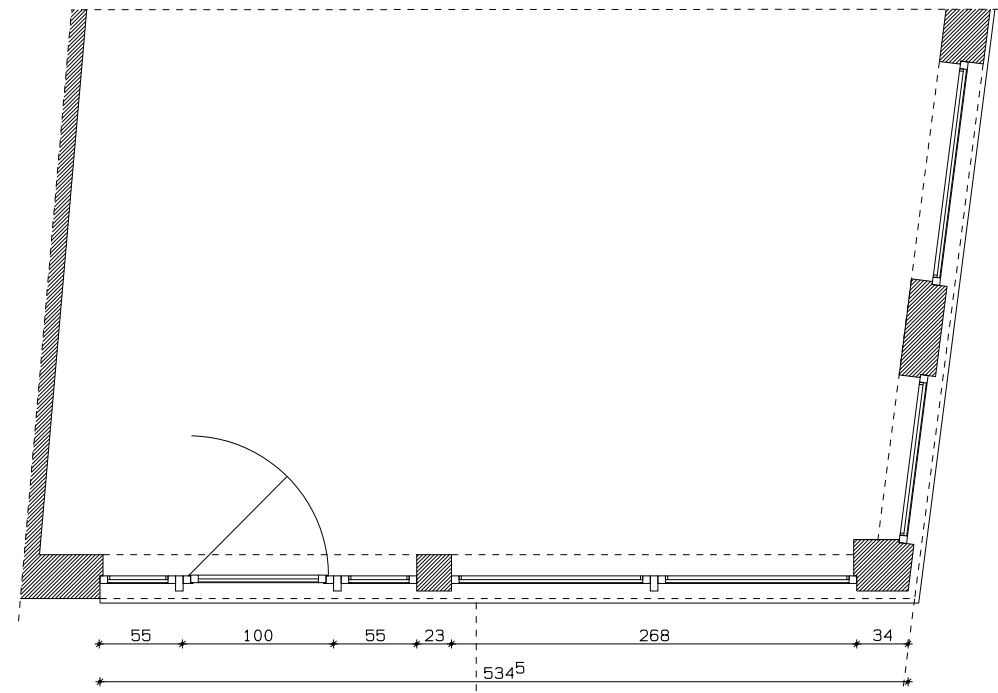
GRONDPLAN VOORGEVEL
