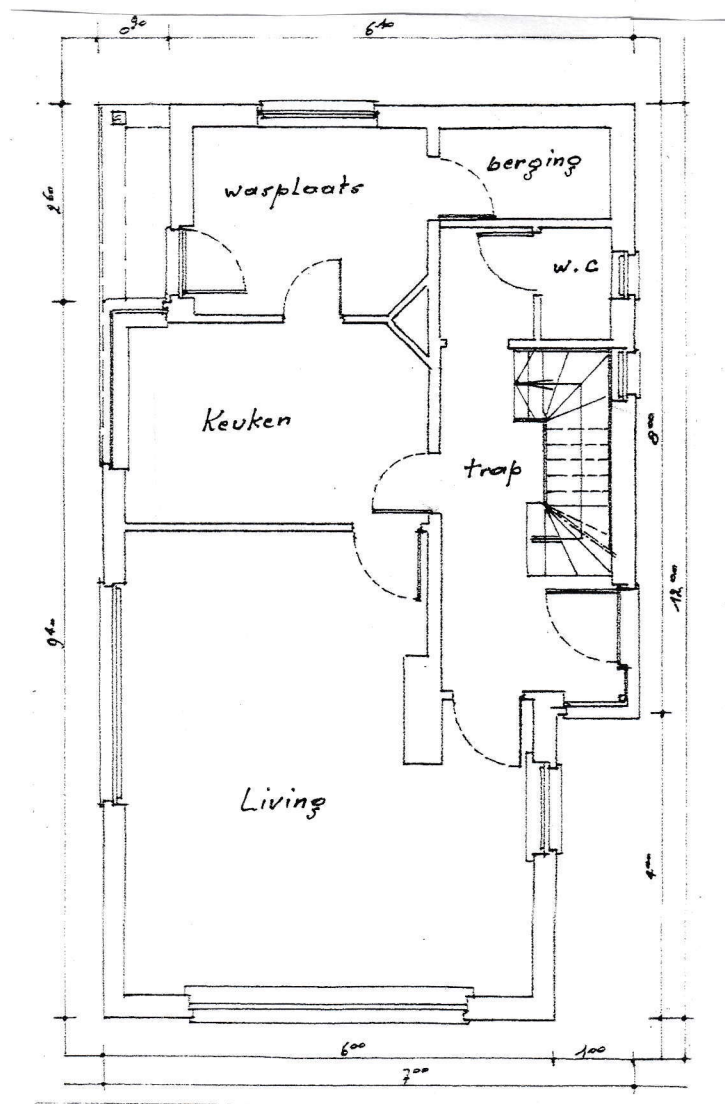
BA_Verbouwen woning met uitbreiding rechter dakkapel_ P_B_01_gelijkvloers schaal /100
