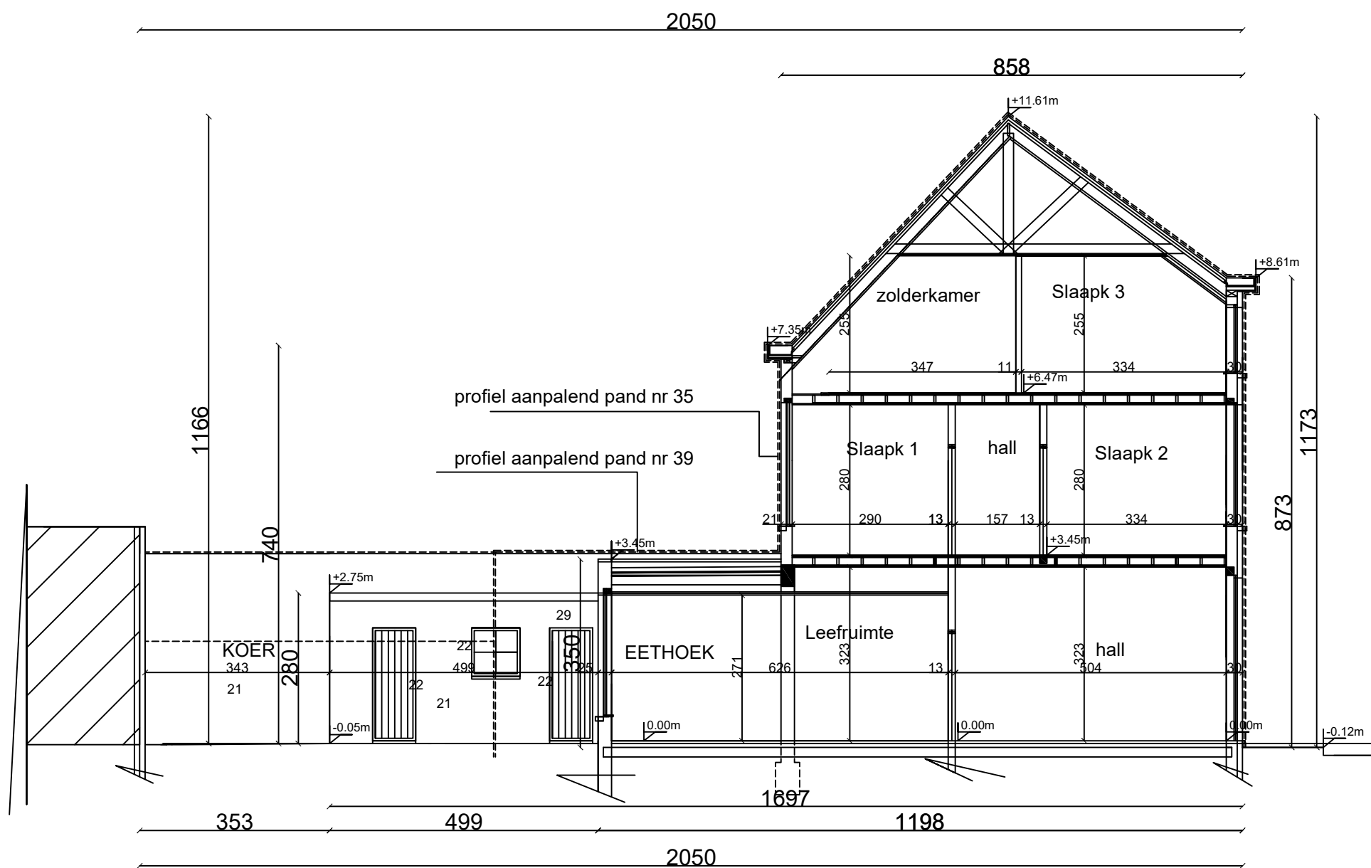
LINKERZIJGEVEL en DOORSNEDE AA' 1/100 Vergunde toestand
