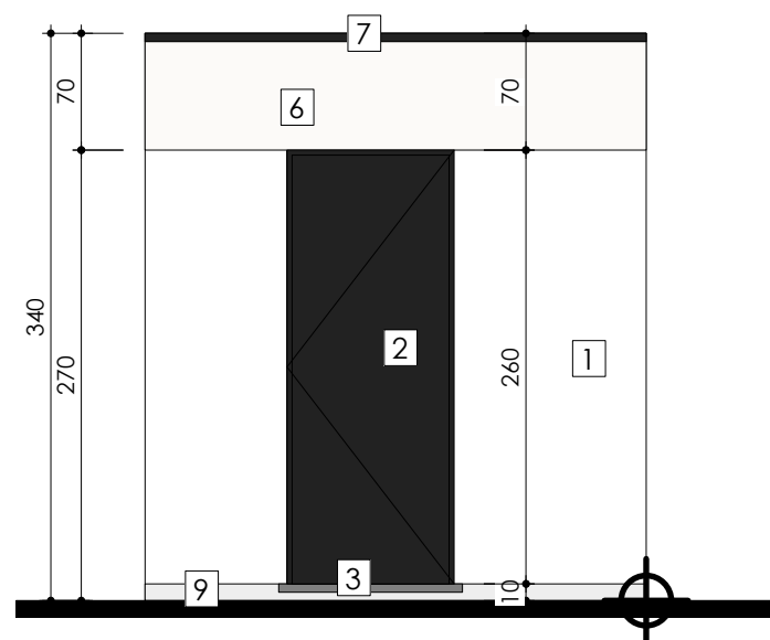
Linker zijgevel - Tuinlounge met tuinberging - Vergunde toestand Schaal: 1:50
