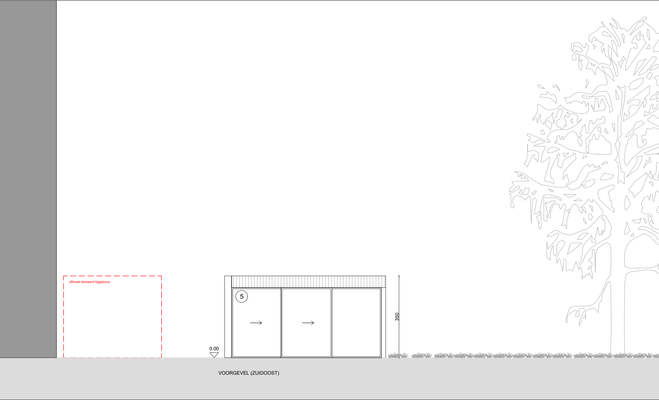
KEIBERG 1 - GENTBRUGGE GEVEL - voorgevel (ZO) vergund
