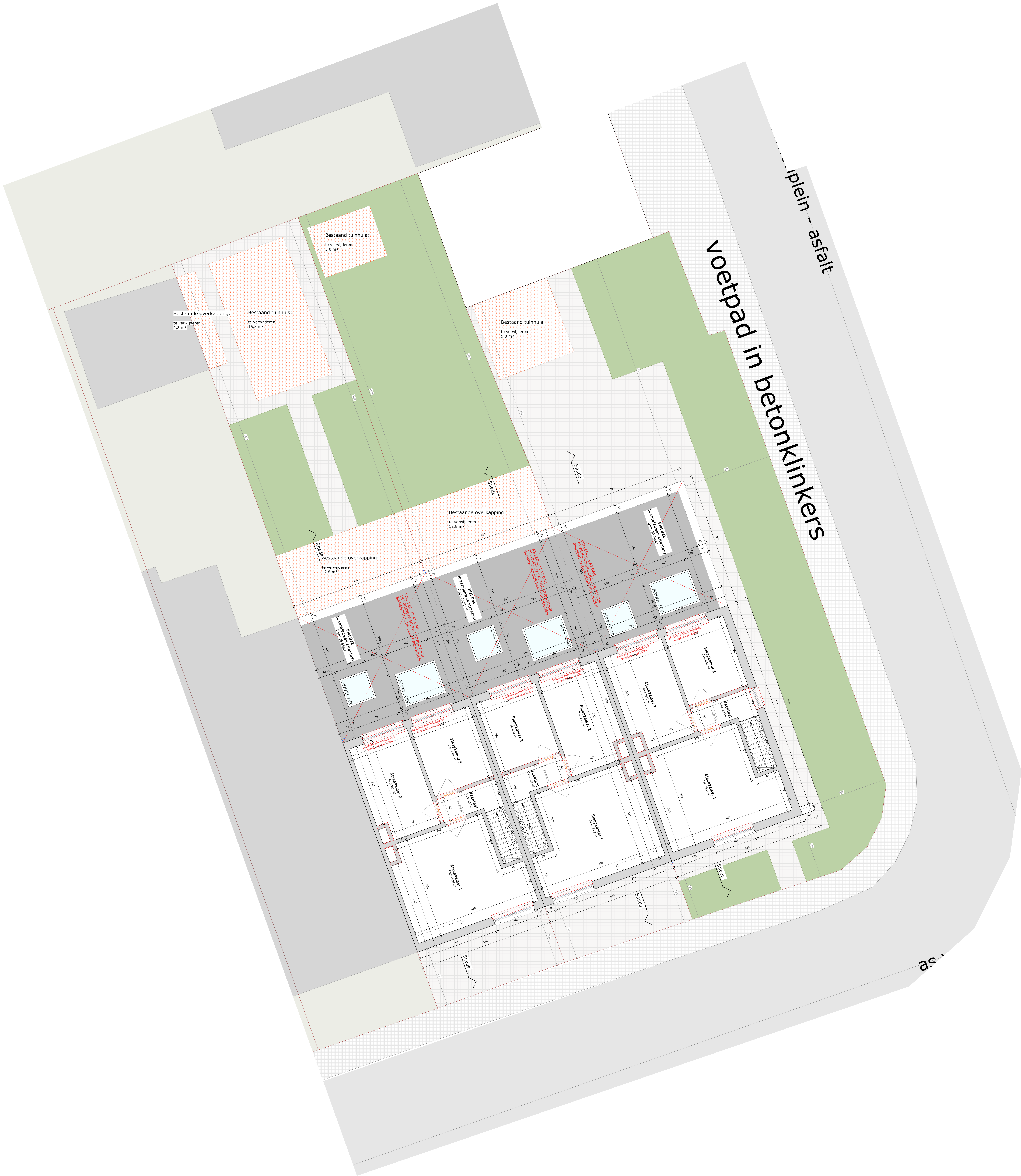
PLAN VERDIEPING 1 - BT schaal 1/50
