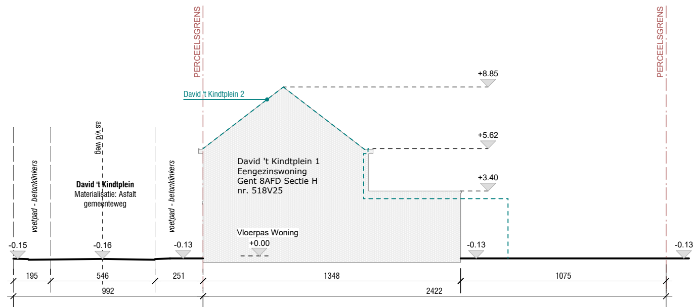
DK 1 - T1 - Terreinprofiel 1 - snede door David 't Kindtplein 1
