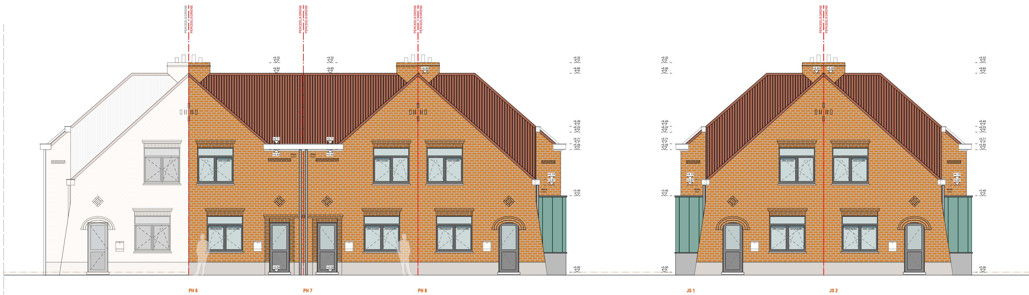
SCHAKELING VOORGEVELS SCHAAL 1/100
