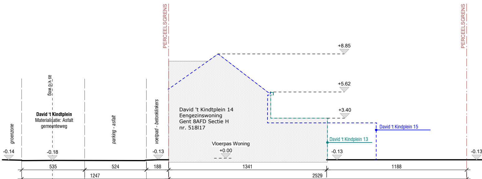
HUB 5 - T4 - Terreinprofiel 4
