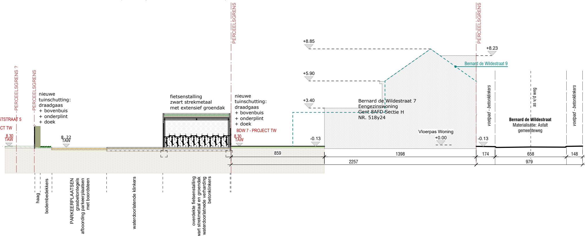
HUB 5 - T1 - Terreinprofiel 1
