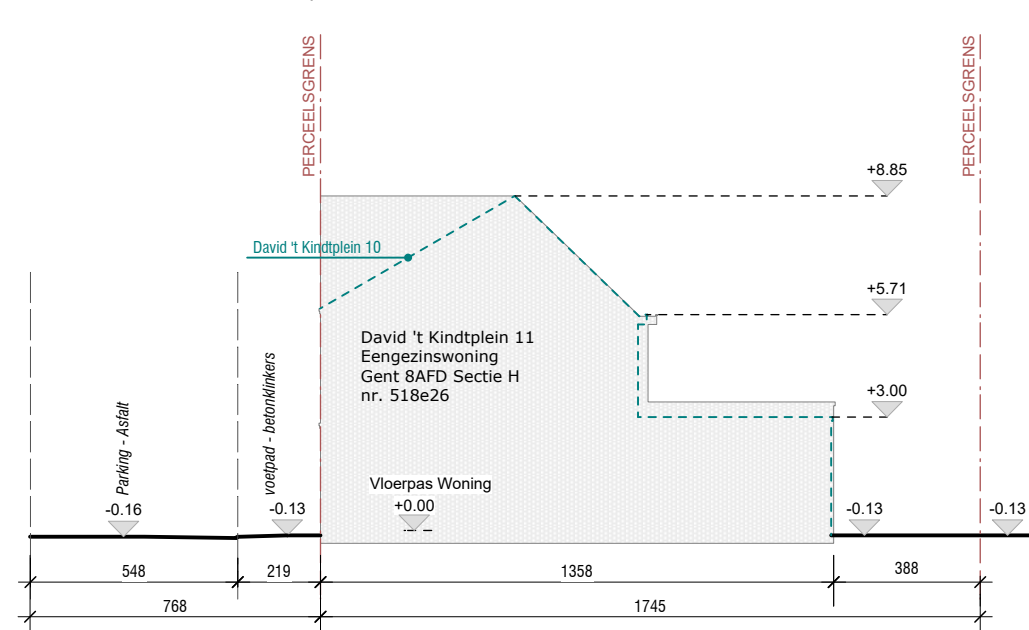
HUB 5 - T5 - Terreinprofiel 5
