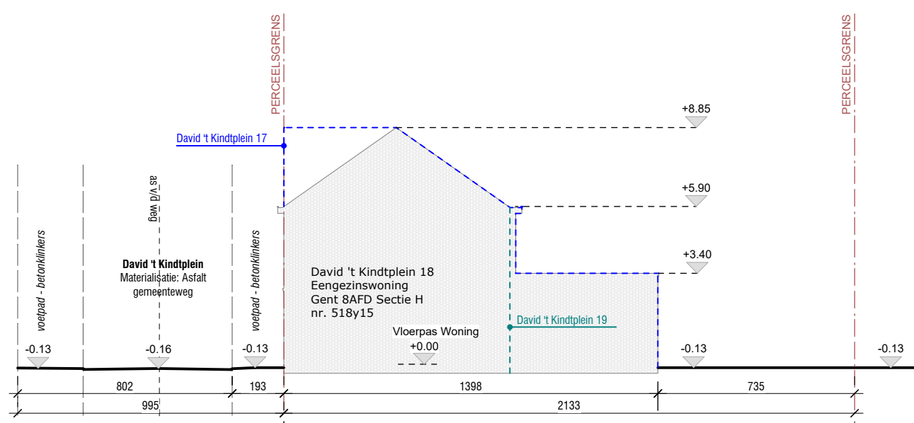
HUB 5 - T3 - Terreinprofiel 3
