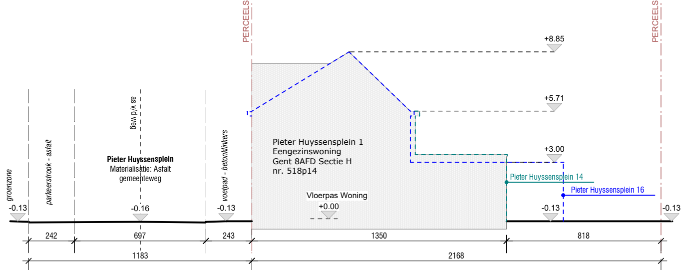
HUB 6 - T4 - Terreinprofiel 4 - snede door Pieter Huyssensplein 15
