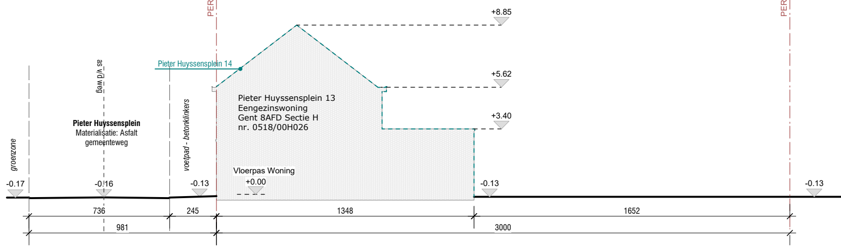
HUB 6 - T3 - Terreinprofiel 3 - snede door Pieter Huyssensplein 13
