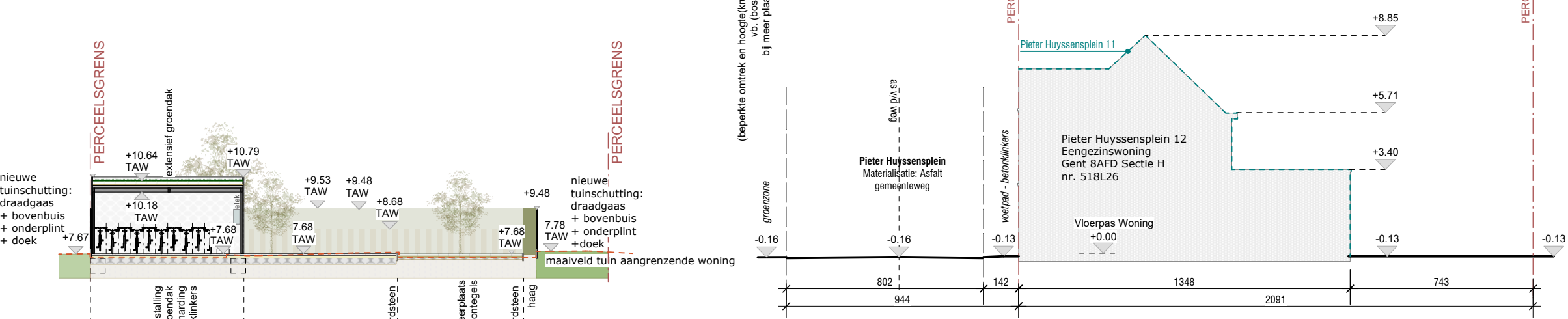
HUB 6 - T5 - Terreinprofiel 5 - snede door Pieter Huyssensplein 12
