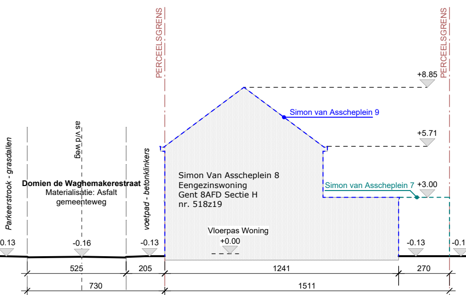
HUB 4 - T4 - Terreinprofiel 4
