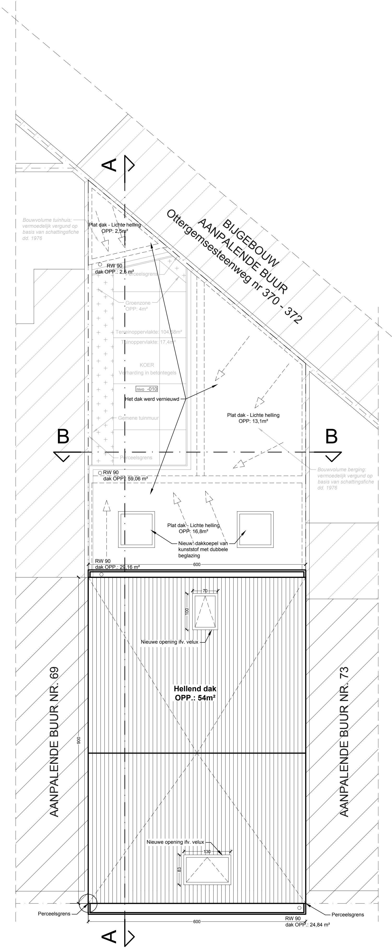
Dakenplan - nieuw = (bestaand)
