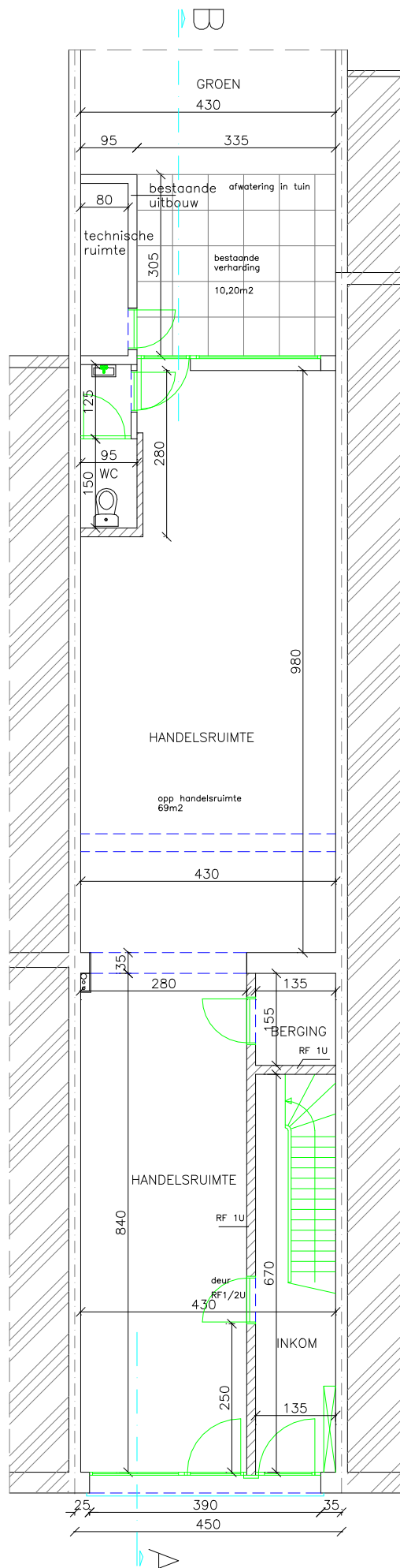
BA woning-P-V-1-gelijkvloers
