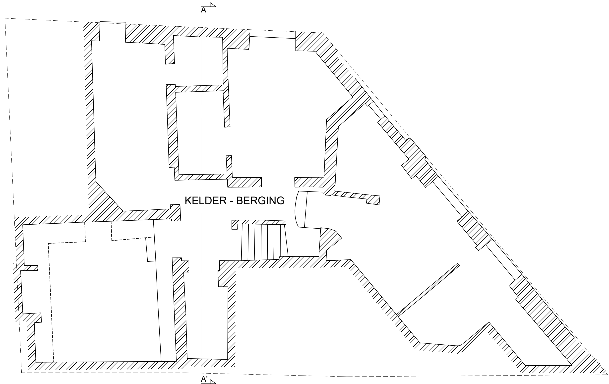
NIV -1 BESTAANDE TOESTAND
